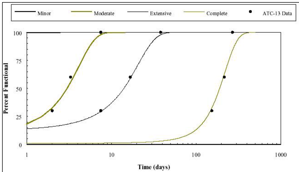
Figura 70. Corbes de restauració per refineries [1].
