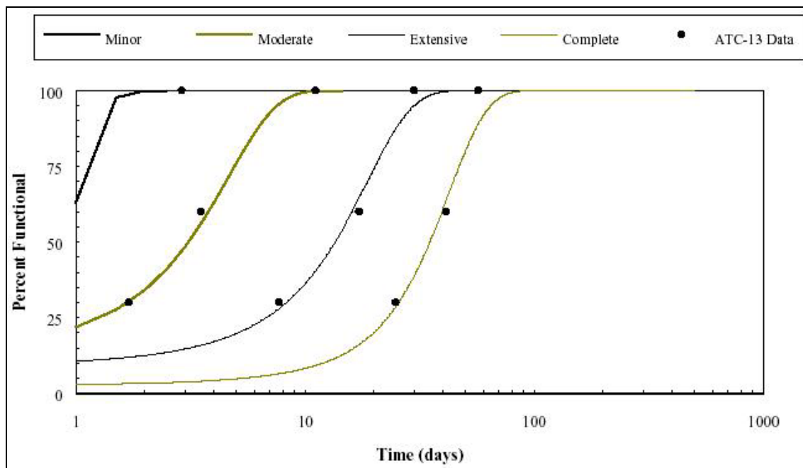
Figura 69. Corbes de restauració per estacions de bombeig [1].
