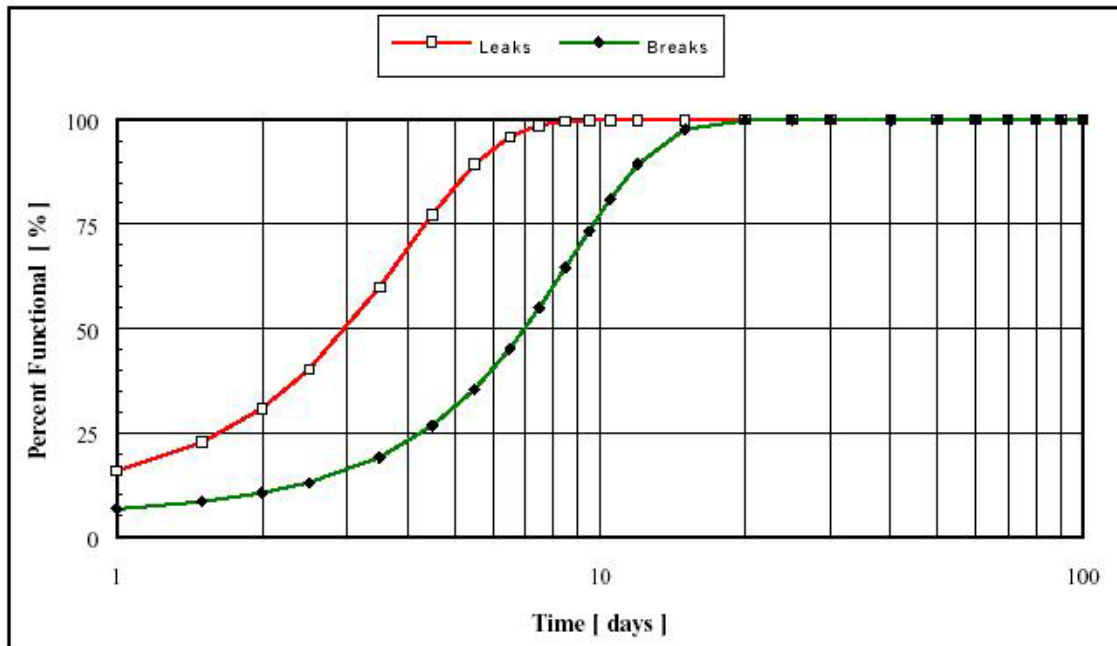
Figura 68. Corbes de restauració per conduccions [1].
