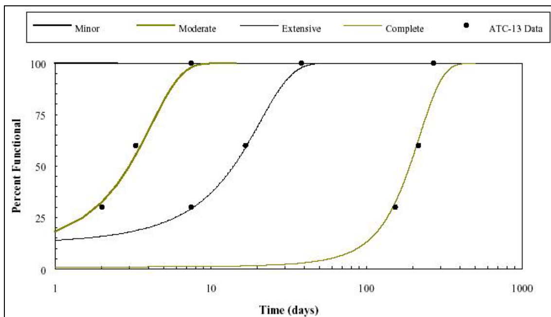
Figura 71. Corbes de restauració per estacions d'emmagatzematge [1].
