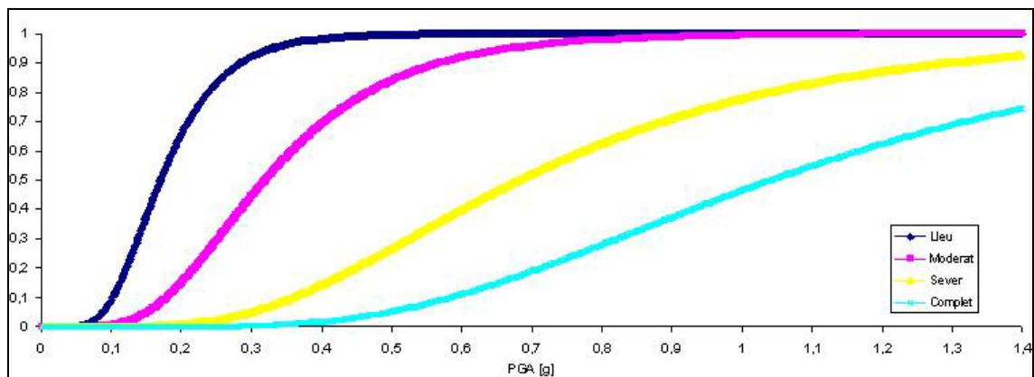
Figura 65. Corbes de fragilitat de les refineries tipus ORF4.
