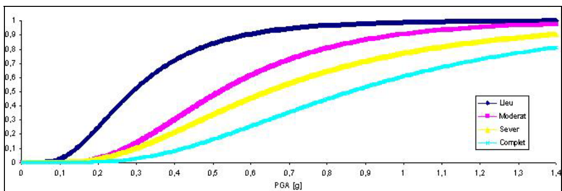
Figura 62. Corbes de fragilitat de les refineries tipus ORF1.
