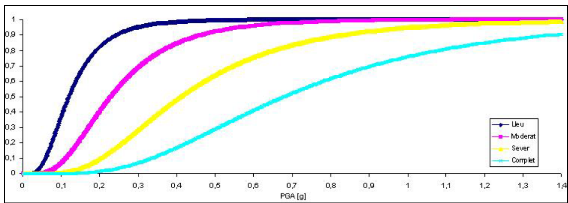
Figura 67. Corbes de fragilitat de les estacions d'emmagatzematge tipus OTF2.
