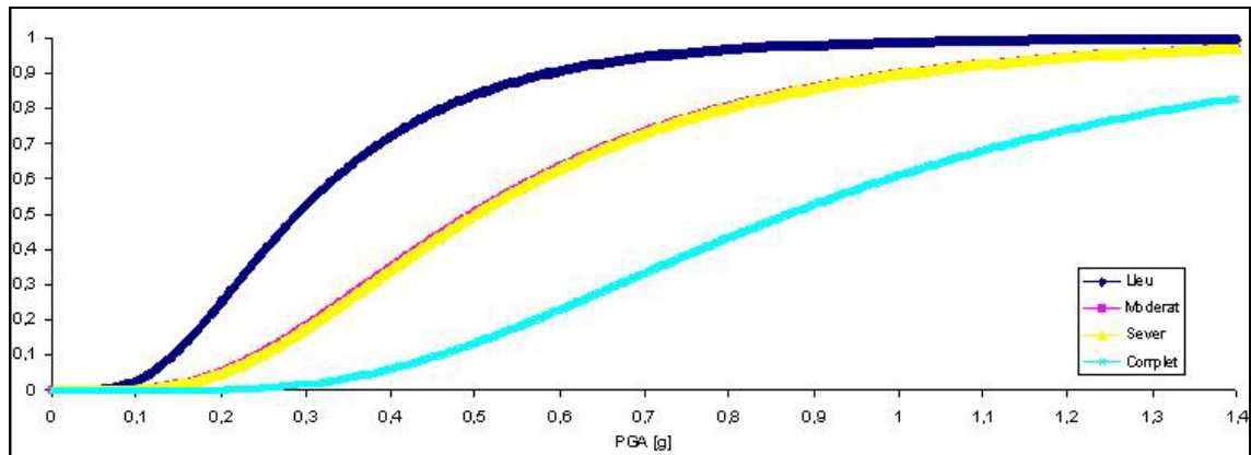
Figura 66. Corbes de fragilitat de les estacions d'emmagatzematge tipus OTF1.
