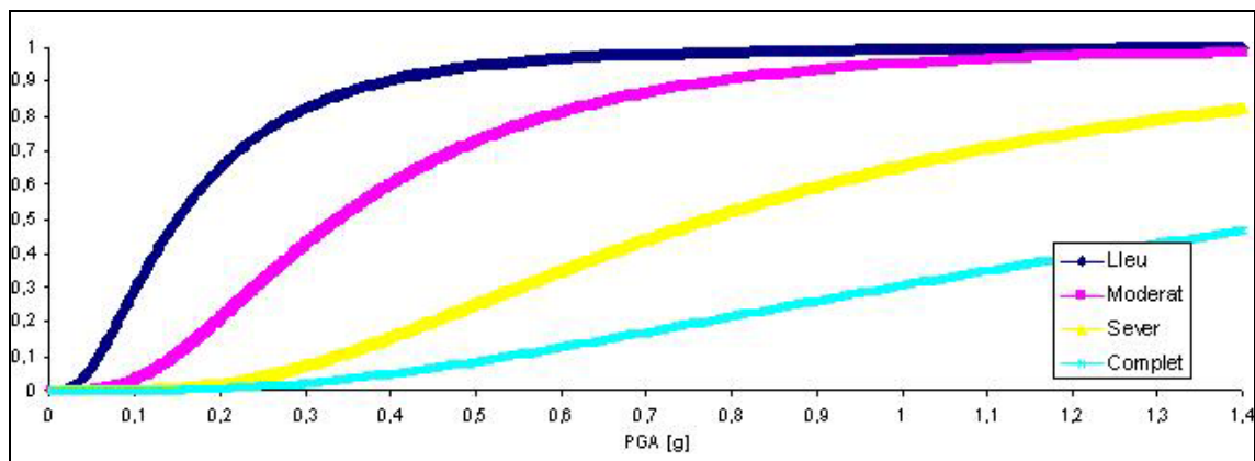
Figura 60. Corbes de fragilitat de les estacions de bombeig tipus OPP1.
