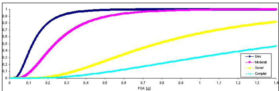
Figura 61. Corbes de fragilitat de les estacions de bombeig tipus OPP2.
