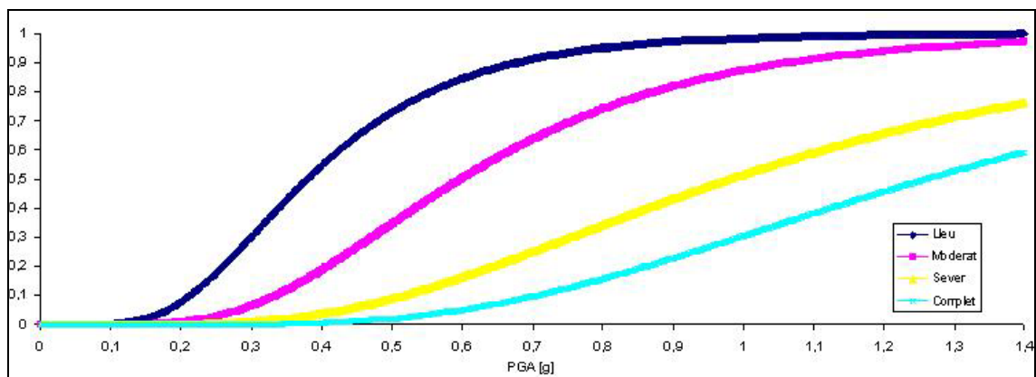
Figura 64. Corbes de fragilitat de les refineries tipus ORF3.
