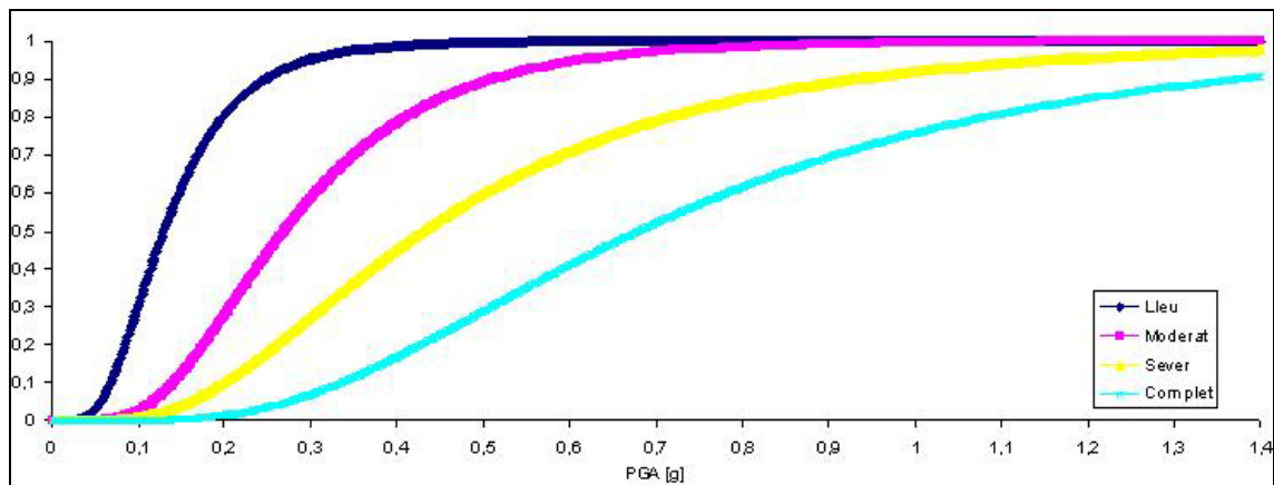
Figura 63. Corbes de fragilitat de les refineries tipus ORF2.
