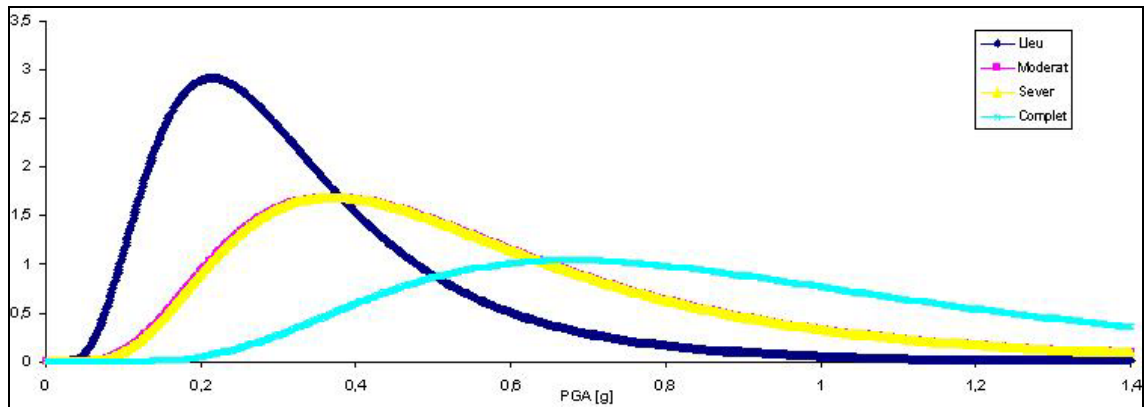
Figura 58. Funcions de densitat de les estacions d'emmagatzematge tipus OTF1.
