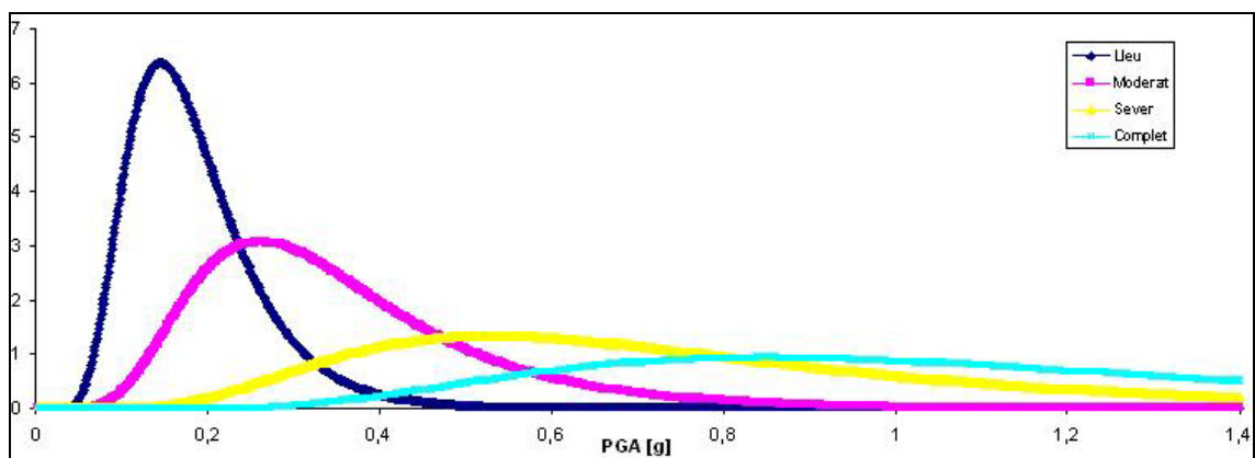
Figura 57. Funcions de densitat de les refineries tipus ORF4.
