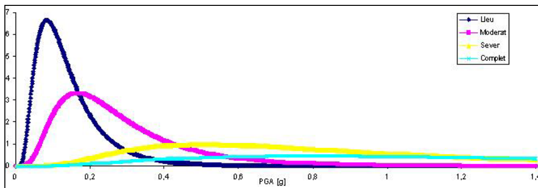
Figura 53. Funcions de densitat de les estacions de bombeig tipus OPP2.
