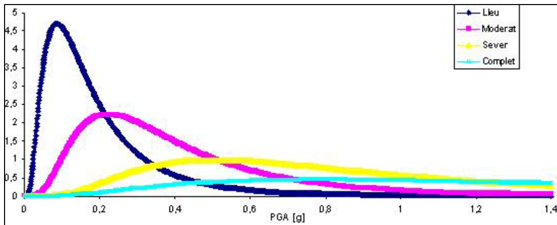
Figura 52. Funcions de densitat de les estacions de bombeig tipus OPP1.
