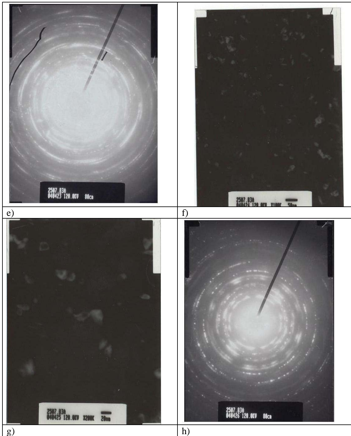
Figura 2. Fotografía y difractograma obtenidos en por TEM en las muestra martensítica
