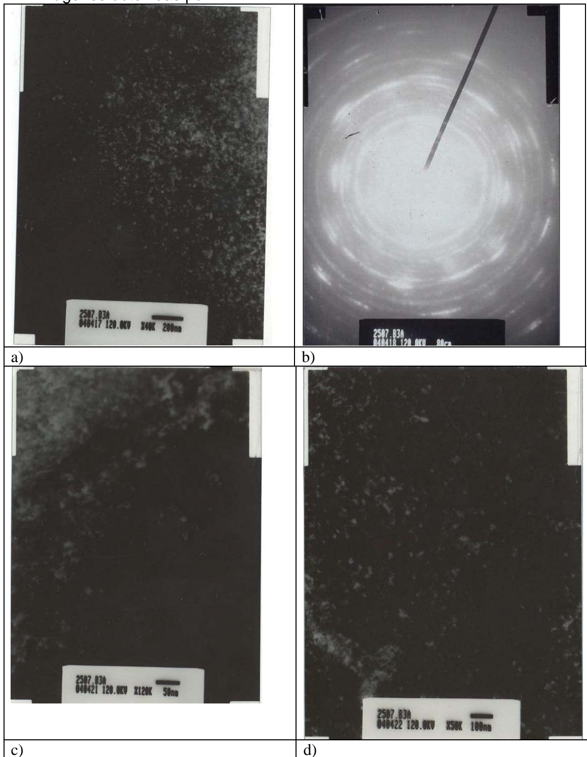
Figura 1. Fotografía y difractograma obtenidos en por TEM en las muestra austenítica
