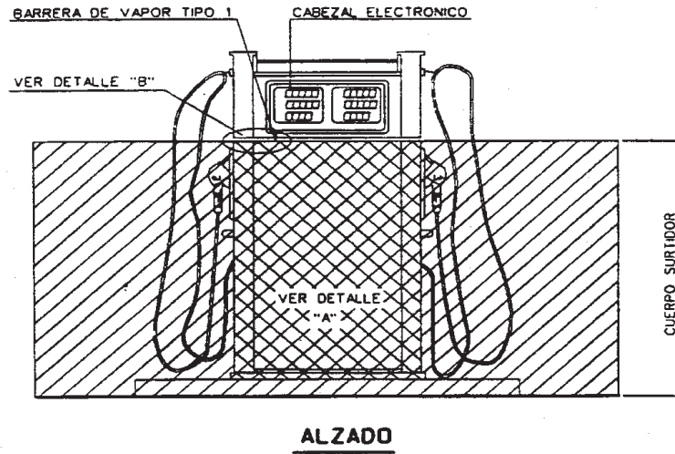
FIG. 1 SURTIDOR CON EL CABEZAL ELECTRÓNICO DIRECTAMENTE MONTADO SOBRE SU CUERPO (BARRERA DE VAPOR TIPO 1)
