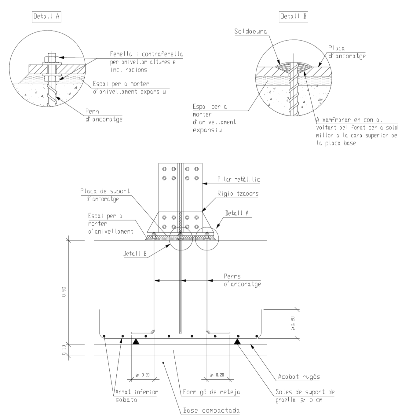
Detall sabota_escalada 1:20
