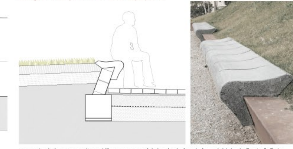
proposta de banc per a l'espai lliure, peça prefabricada de formigó model fola de Sarda & Cole col·locat sobre muret armat de blocs de formigó, revestit amb una xapa d'acer contún
