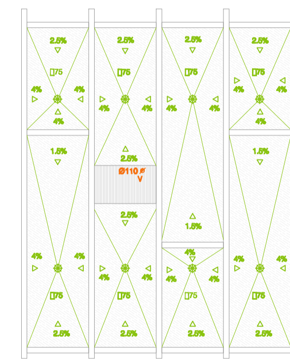
PLANTA SEGONA SOSTRE DESGUÀS - COL-LECTORS PENJATS E/1:200
