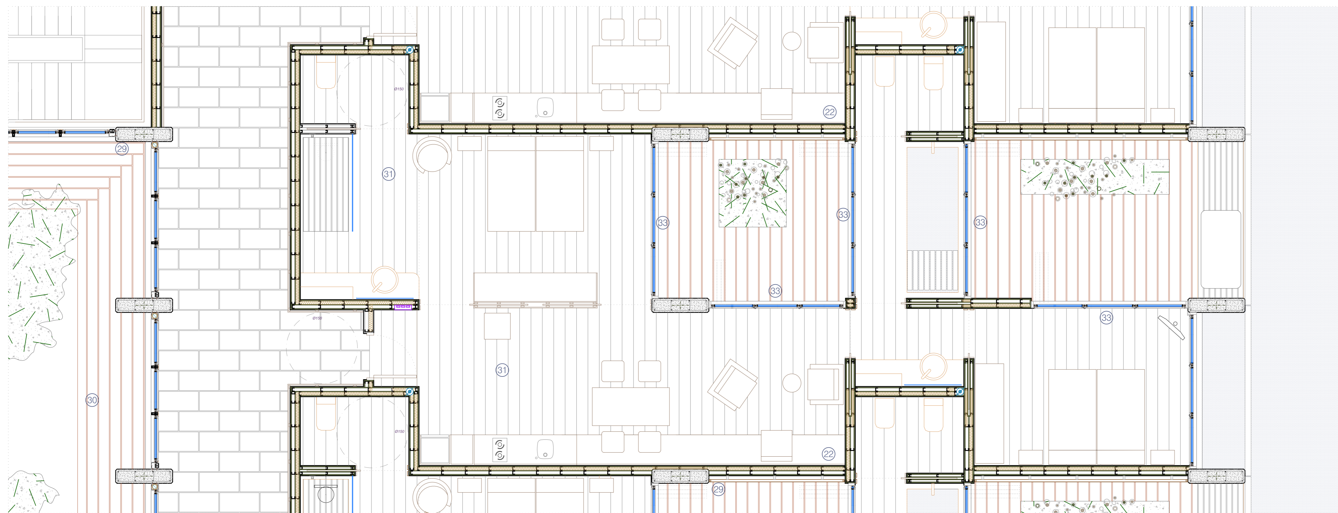
PLANTA ZONA APARTAMENTS P.BAIXA e:1/50
