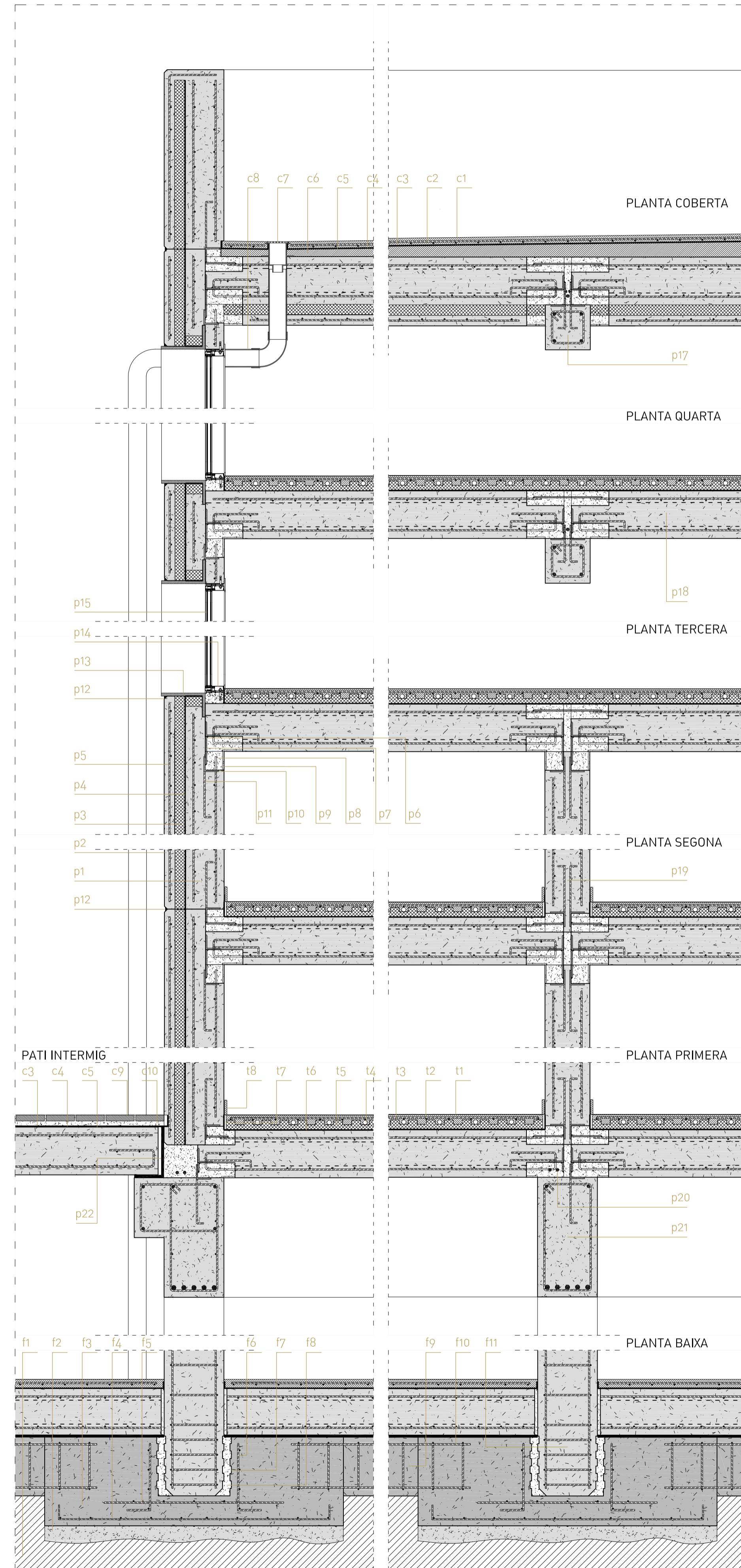
SECCIÓ B-B'
