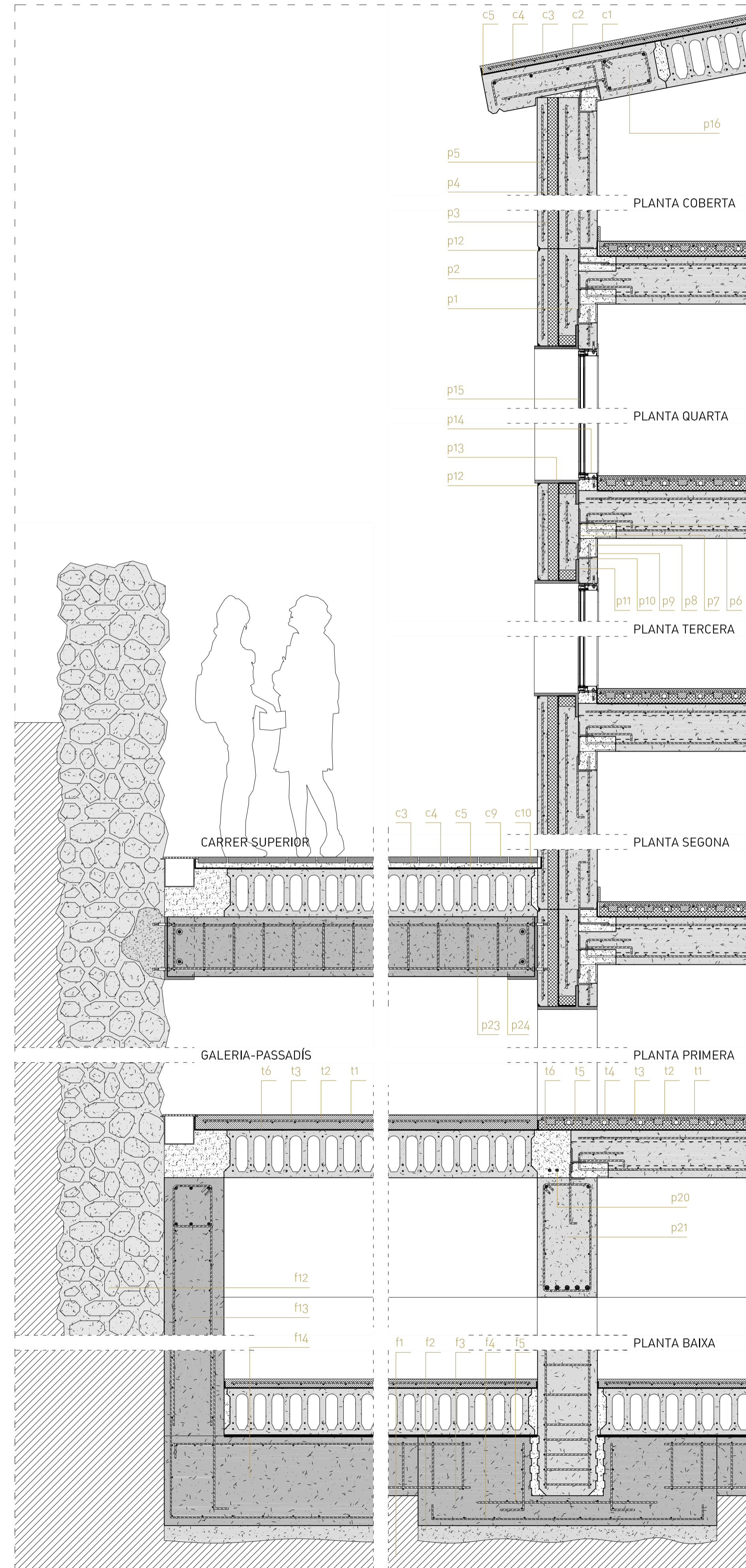
SECCIÓ A-A'
