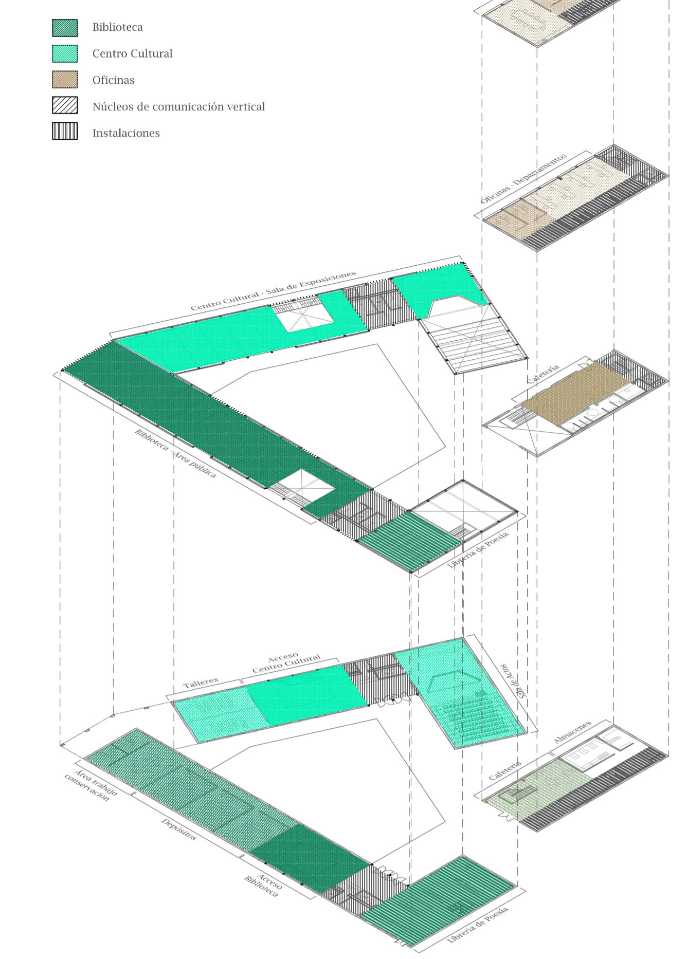
Distribución del programa e. 1/500
