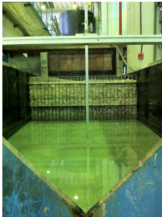
(d) Detalle del vertedero triangular.
