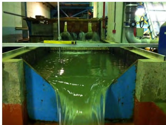
(e) Vertedero triangular en funcionamiento.
