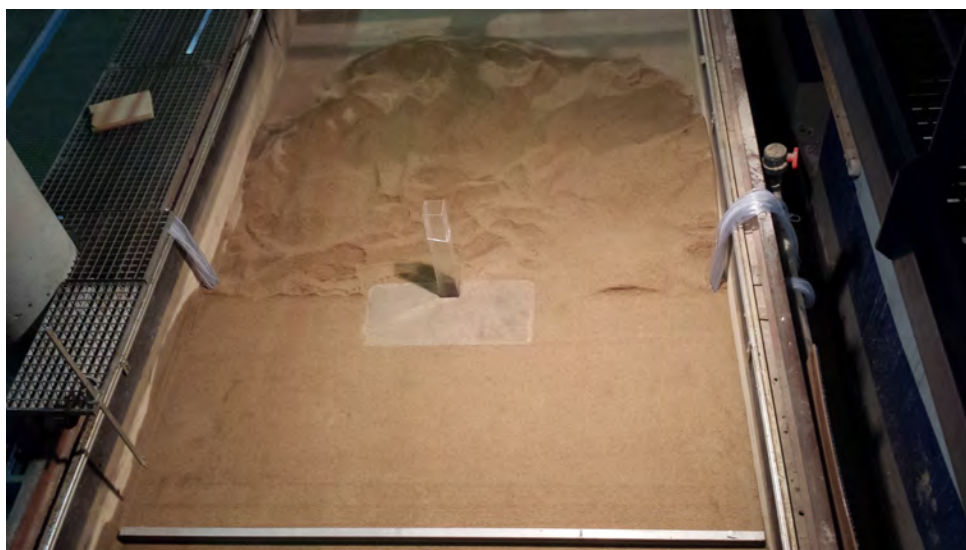
(d) Enrasado de la arena.
