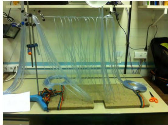
(d) Montaje de los tubos en la piedra.
