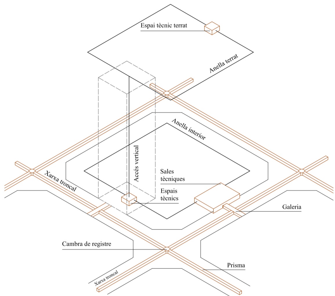
SISTEMES DE CLIMATITZACIÓ Esquema de la xarxa de climatització en superilles 1/2000
