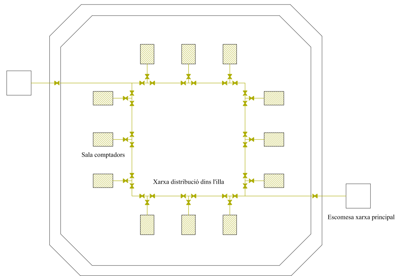
SUBMINISTRAMENT DE GAS Distribució dins d'una illa 1/1000
