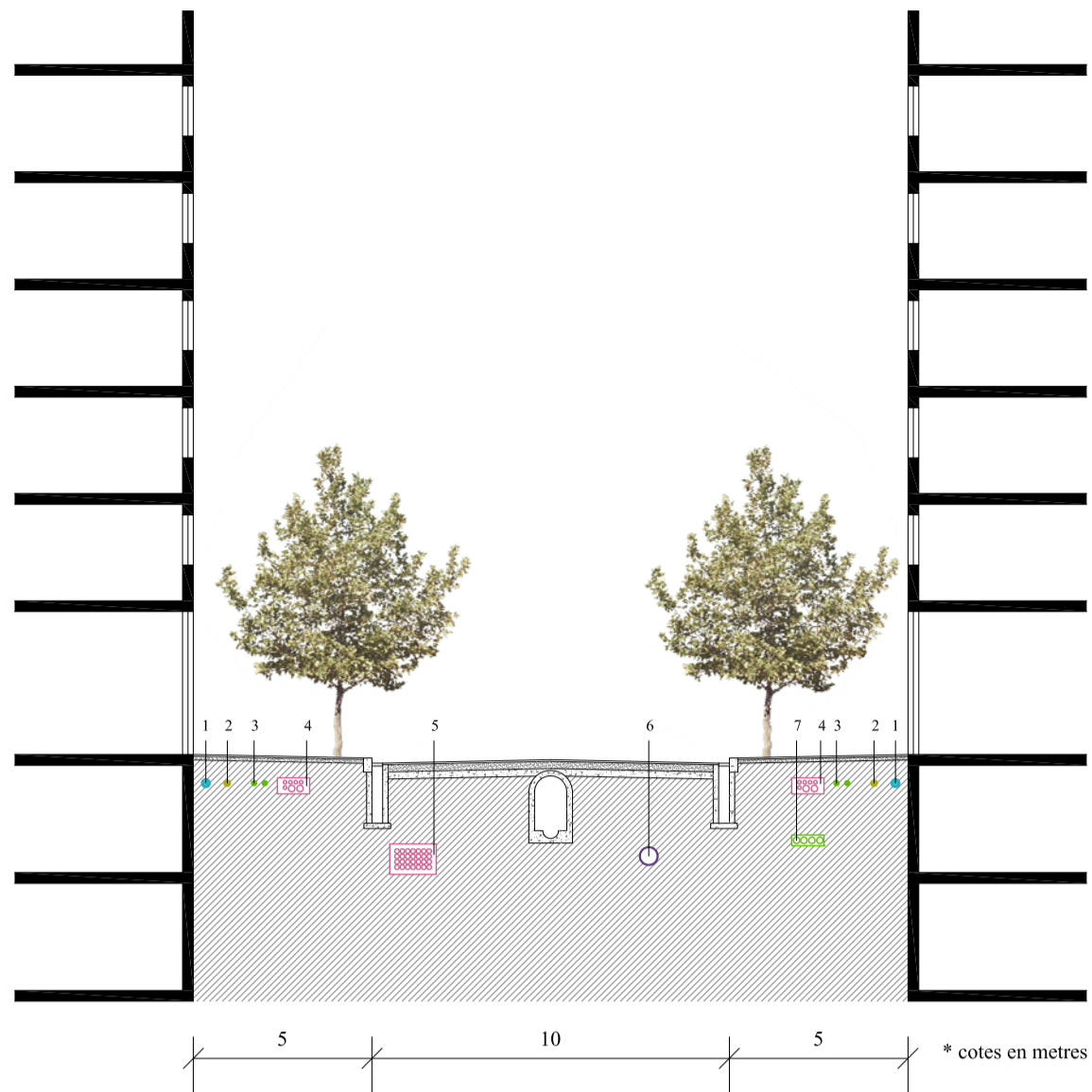
CARRER DE CRISTÓBAL DE MOURA Secció tipus de subsòl 1/200
