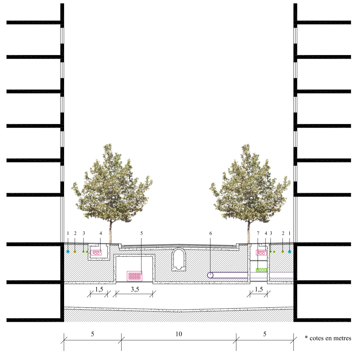
CARRER DE CRISTÓBAL DE MOURA Secció tipus de subsòl amb galeria de serveis 1/200
