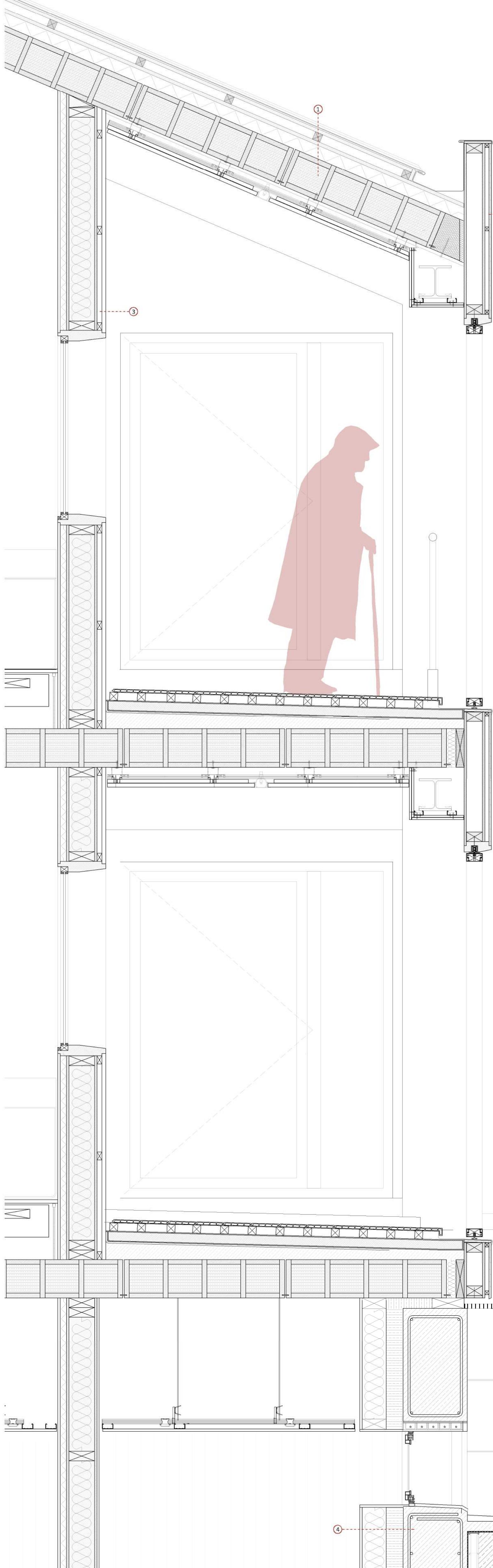
SECCIÓ DETALL FAÇANA PAVELLÓ TIPUS 1:15
