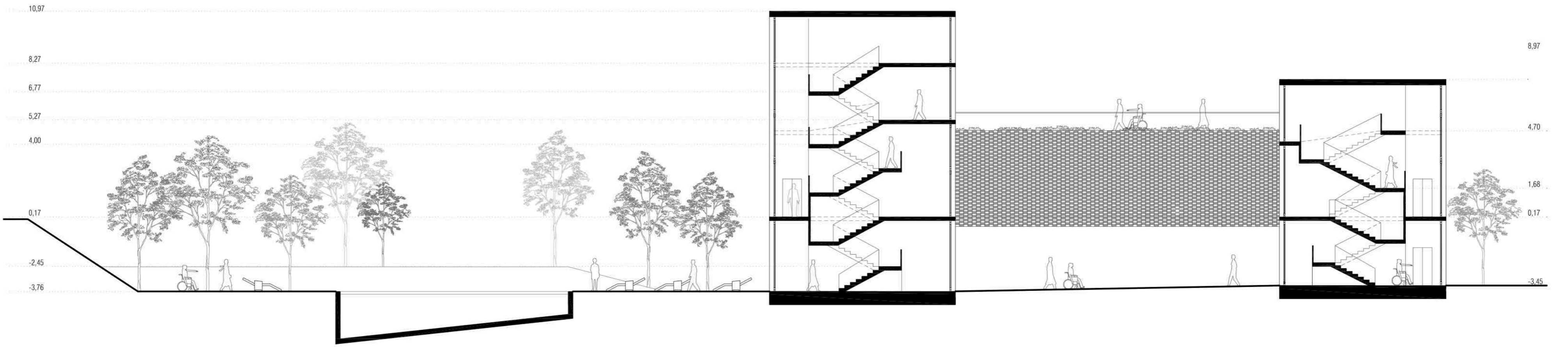
SECCIÓN 1T
