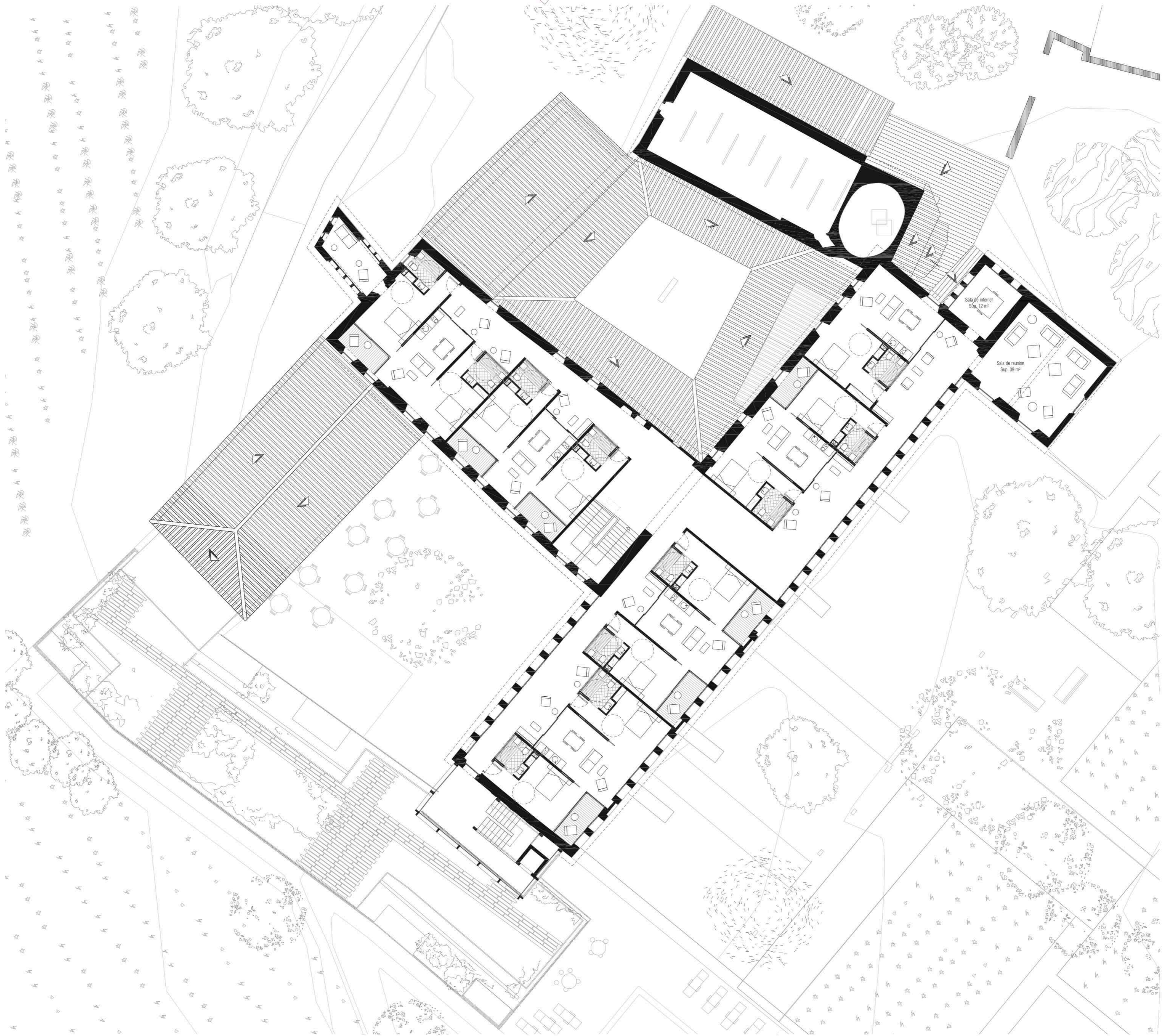
PLANTA +2
