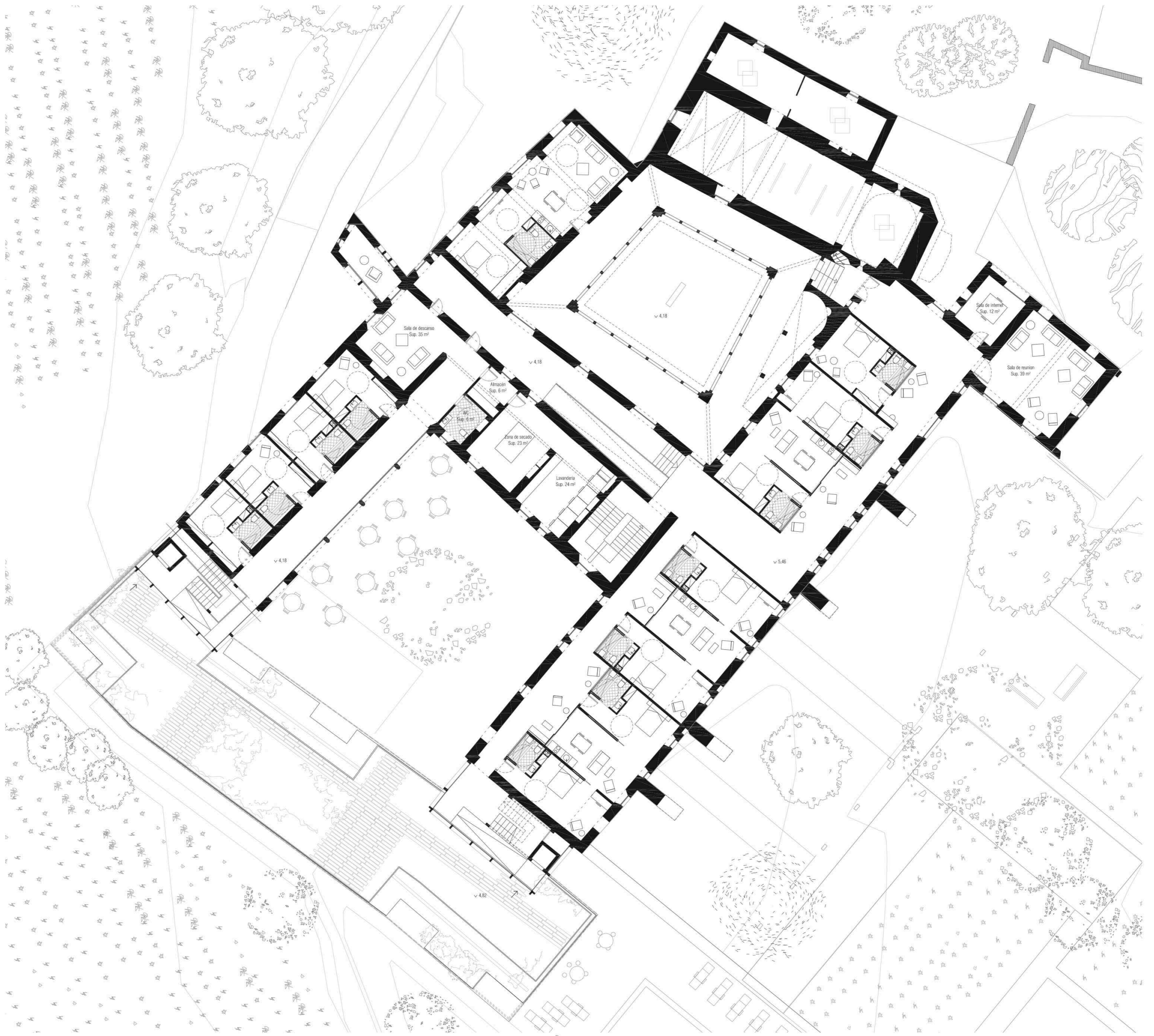
PLANTA +1
