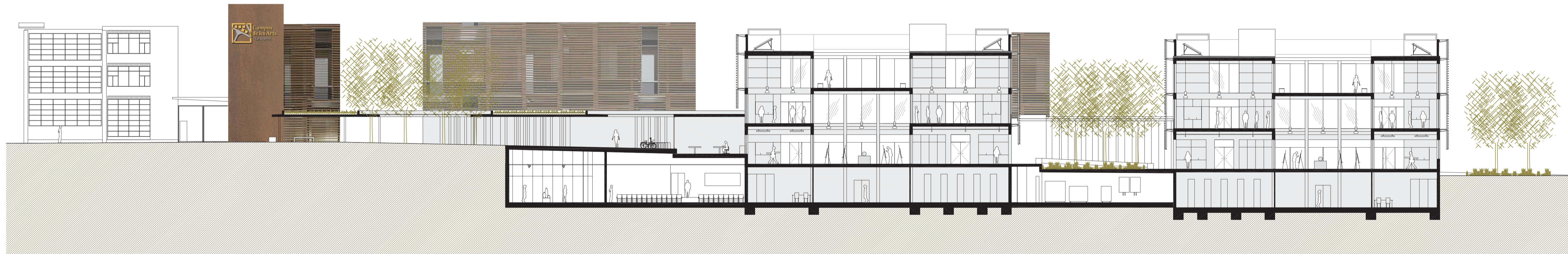
S2_SECCIÓ LONGITUDINAL (A TRAVÉS DEL MÒDUL)
