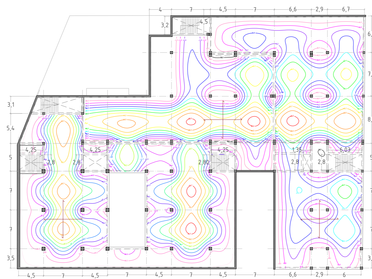
Isolinies sostre psot e. 1/400
