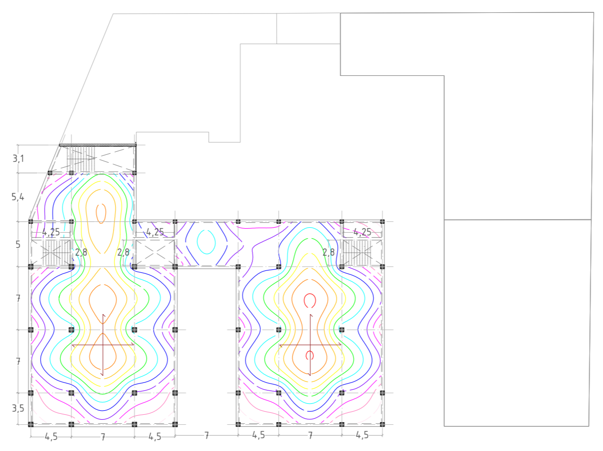
Isolinies sostre p4 e. 1/400
