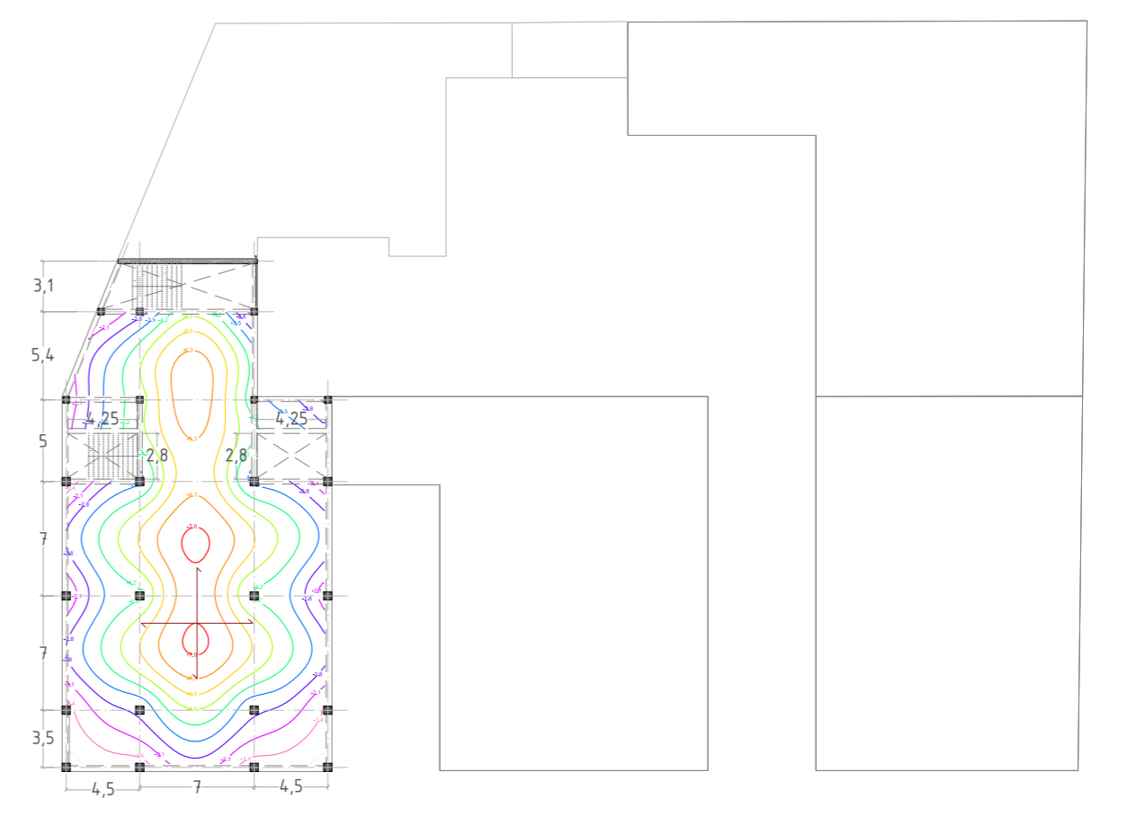
Isolinies sostre p6 e. 1/400
