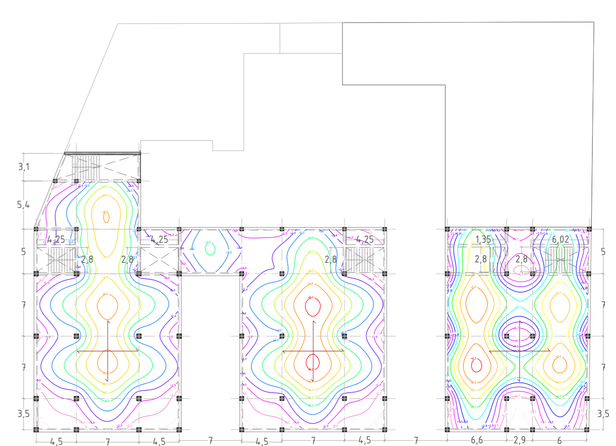
Isolinies sostre p2 e. 1/400
