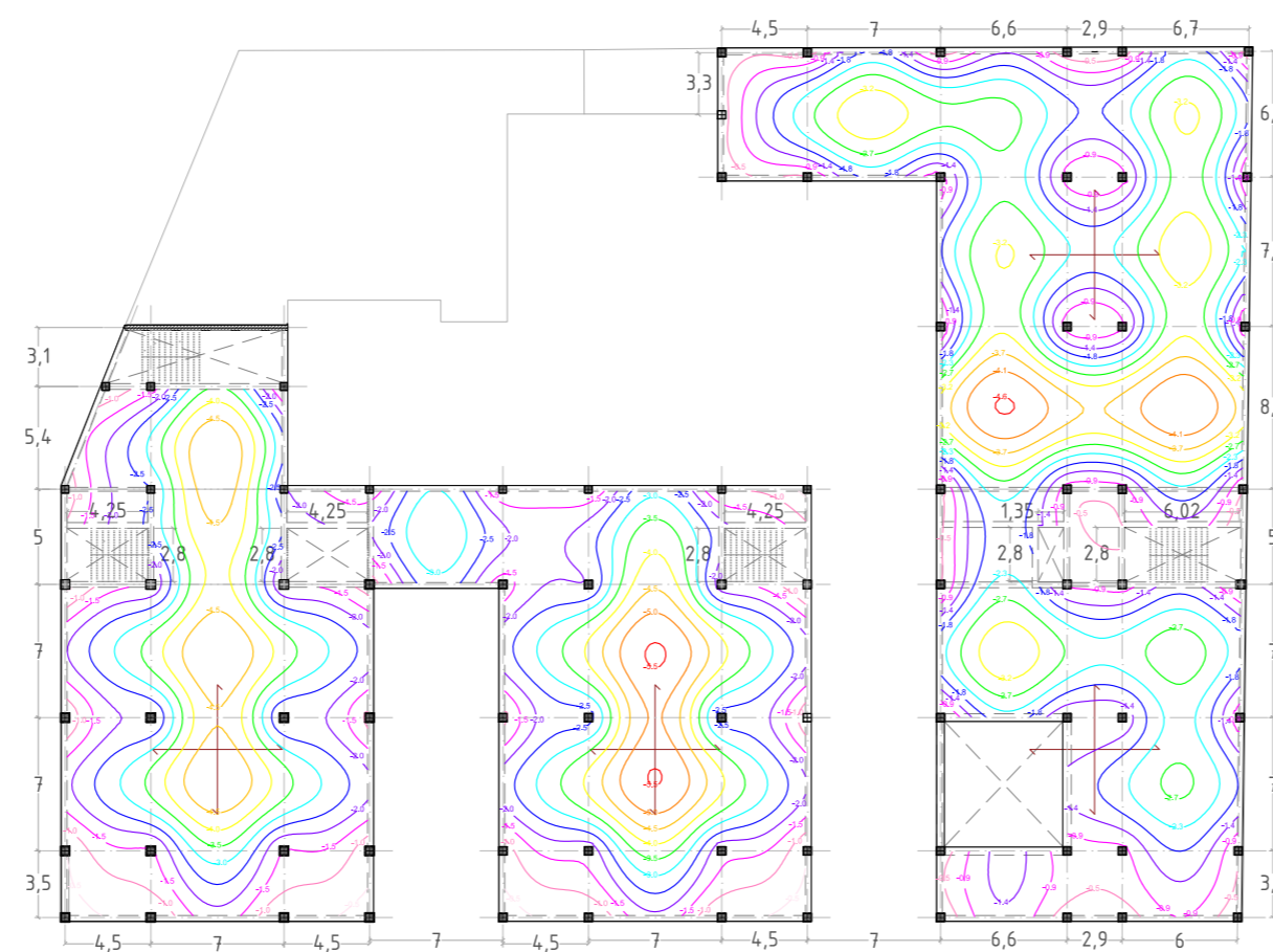
Isolinies sostre p1 e. 1/400
