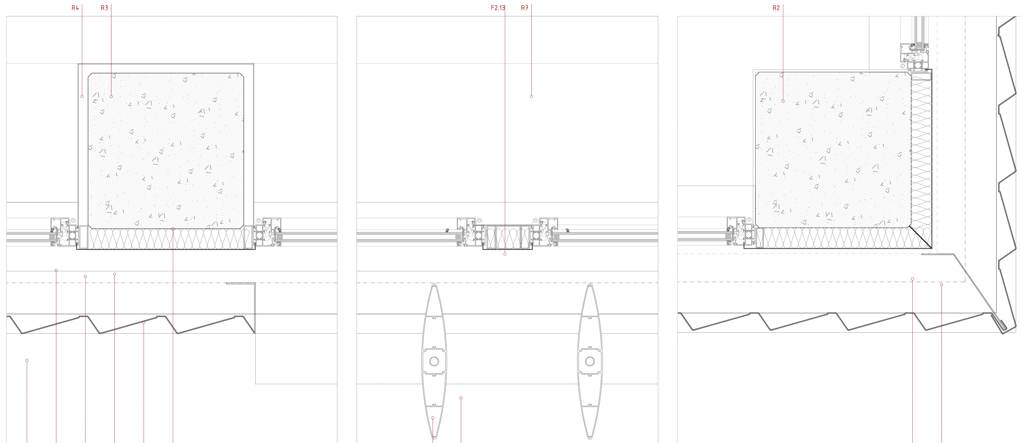
Secció horitzontal e. 1/20
