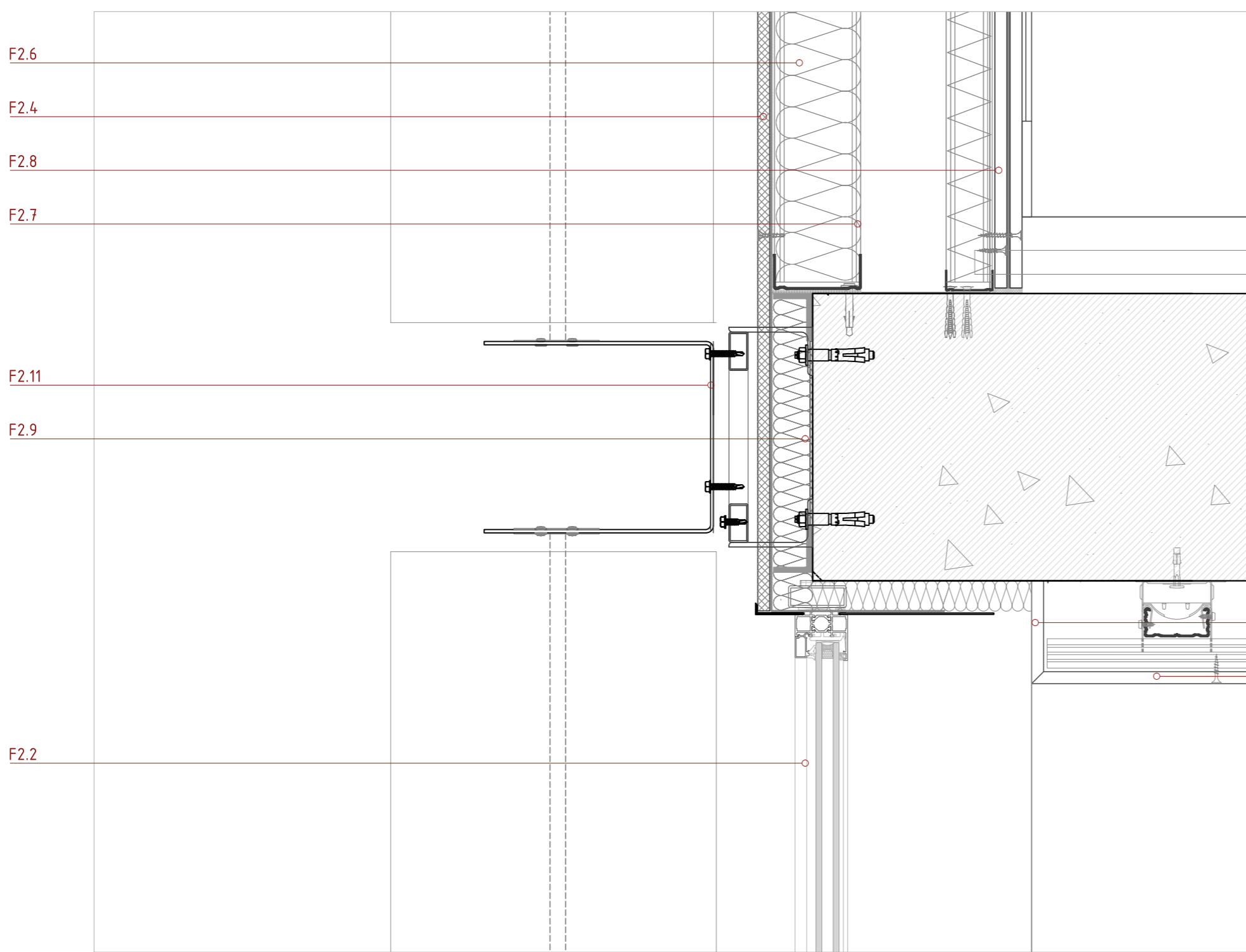
Detall D02 e. 1/5
