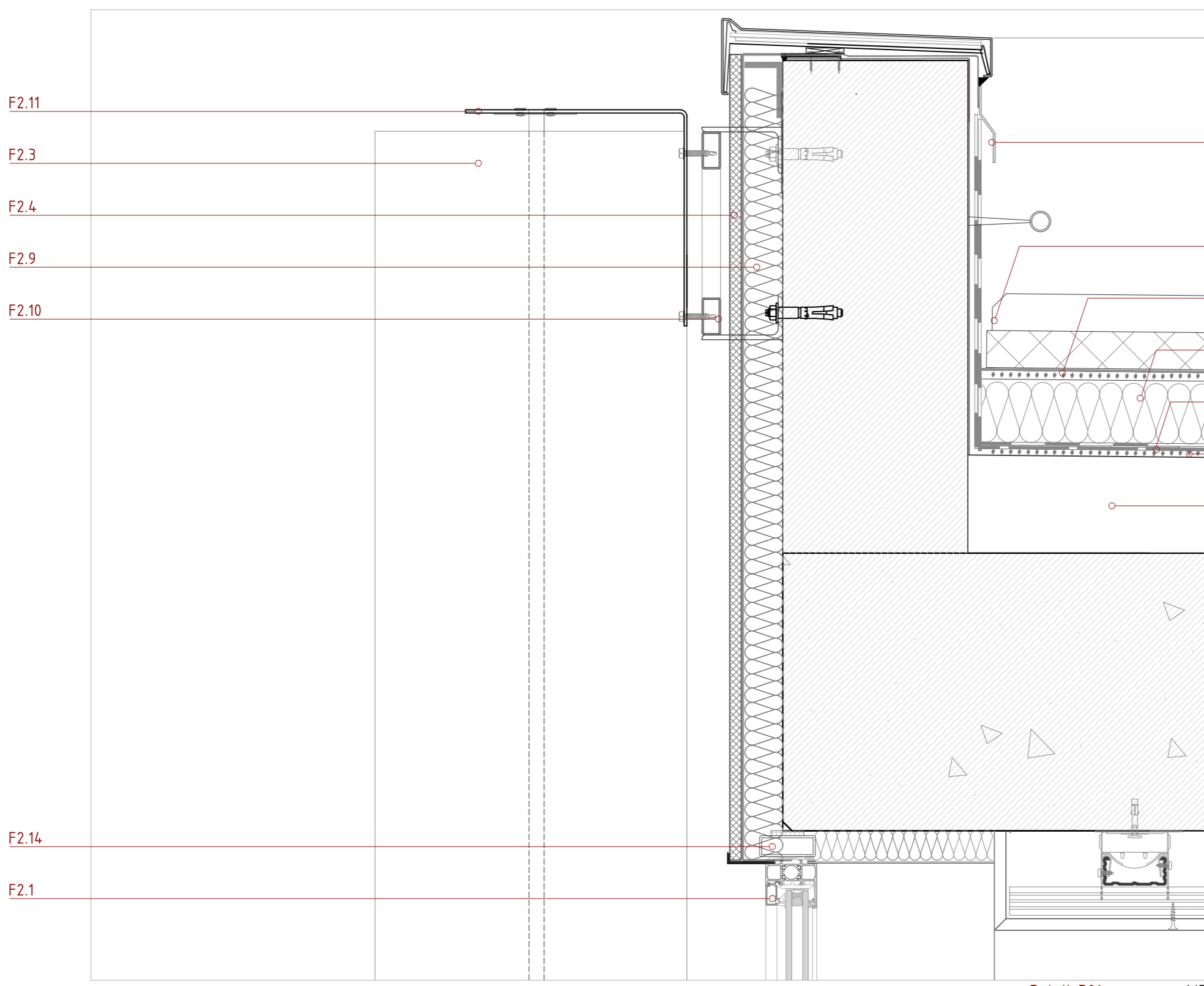
Detall D01 e. 1/5
