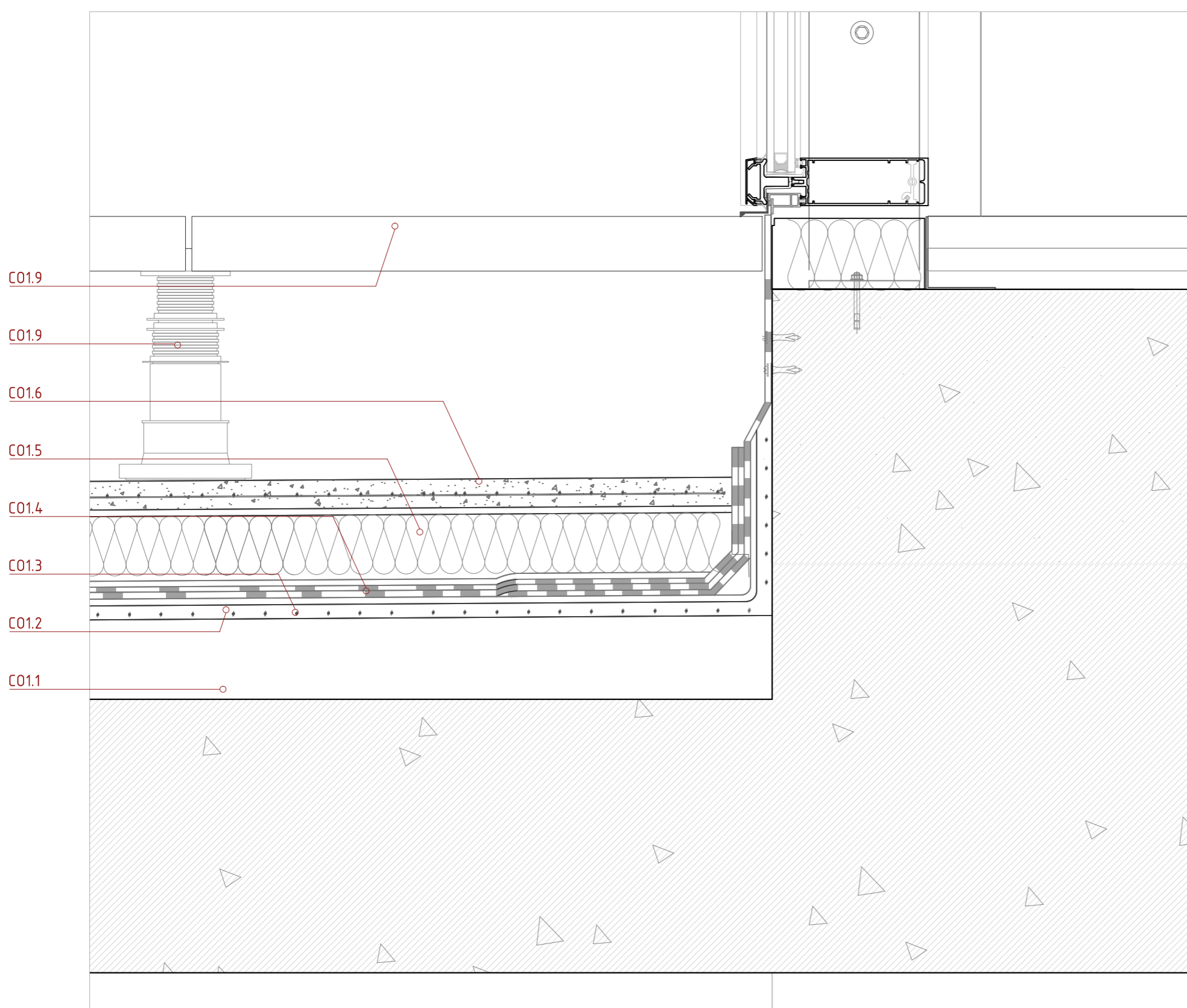
Detall D04 e. 1/5
