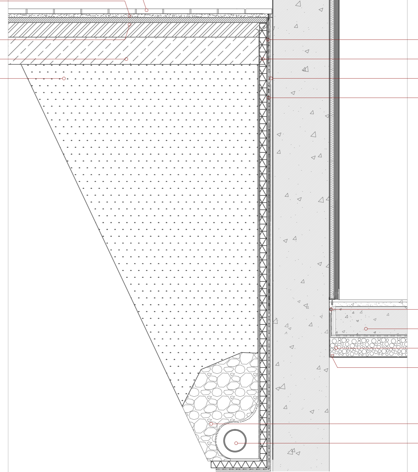
Secció vertical e. 1/20
