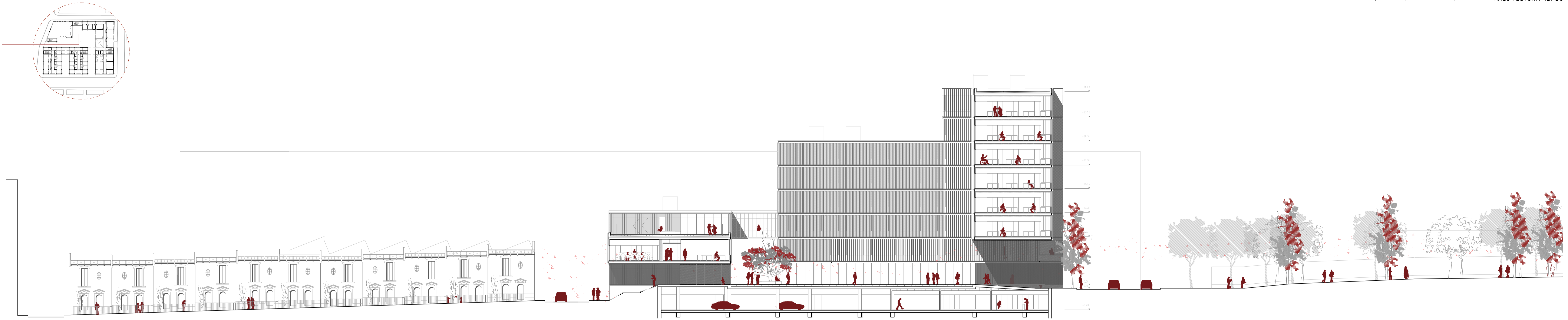
Secció 1 e. 1/200
