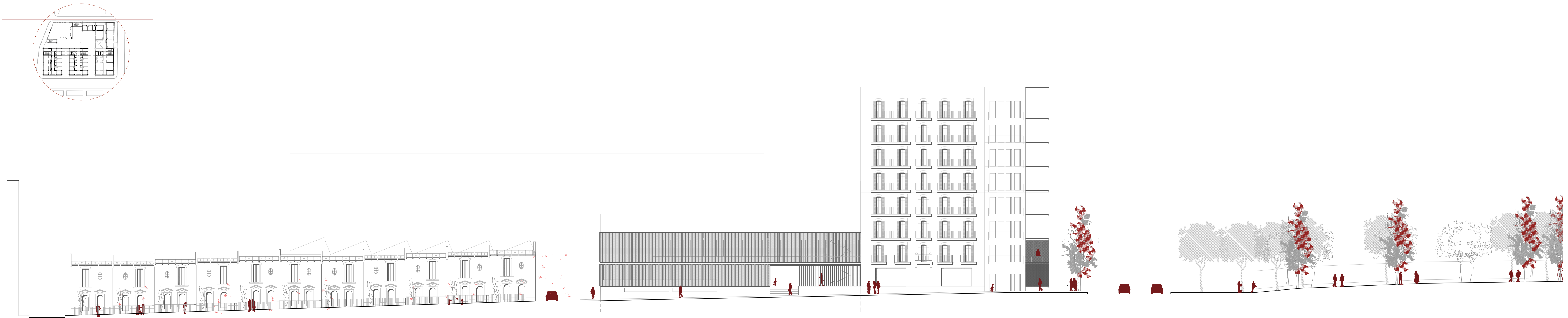
Secció 1 e. 1/200
