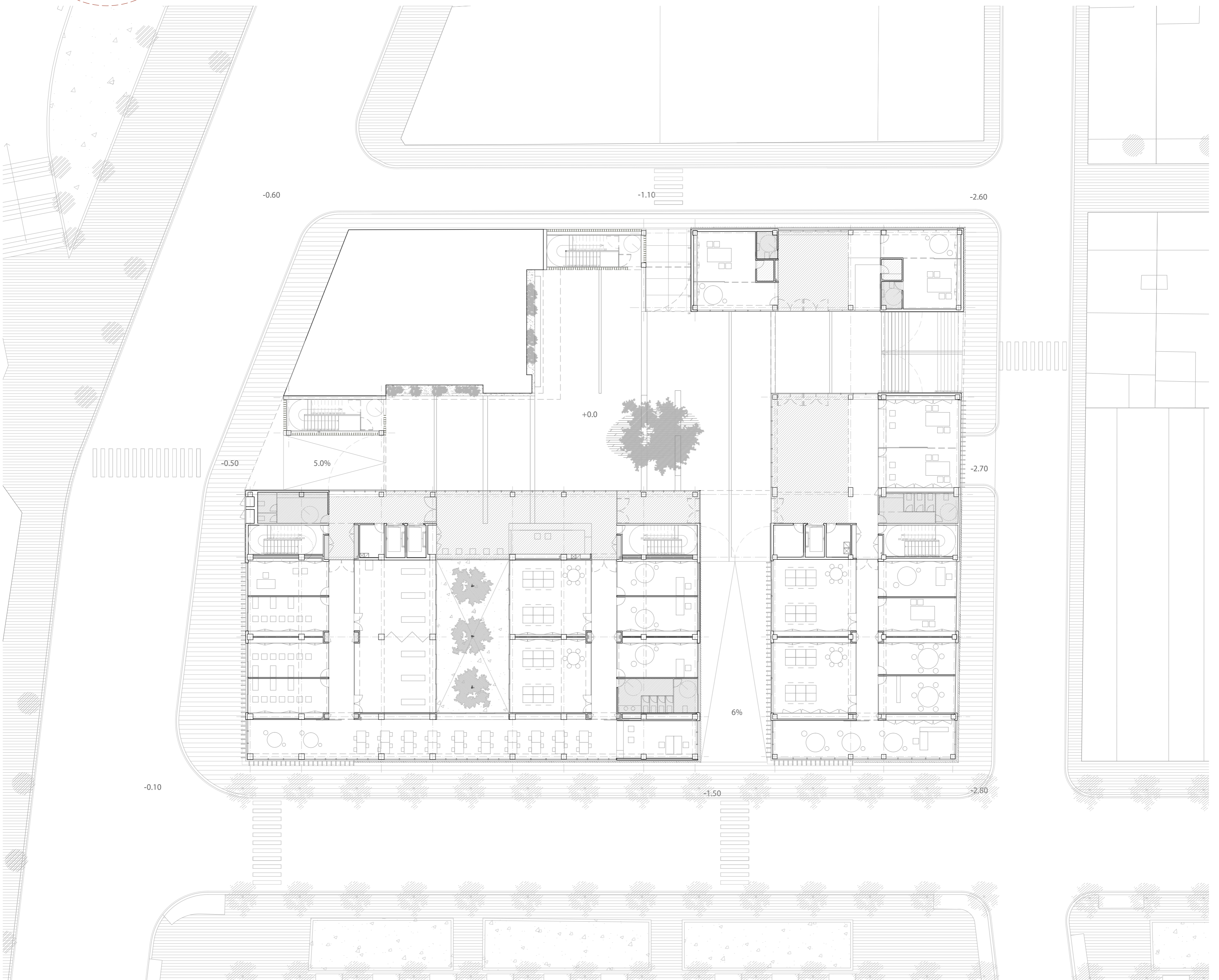
Planta pb ( -0,0m)
