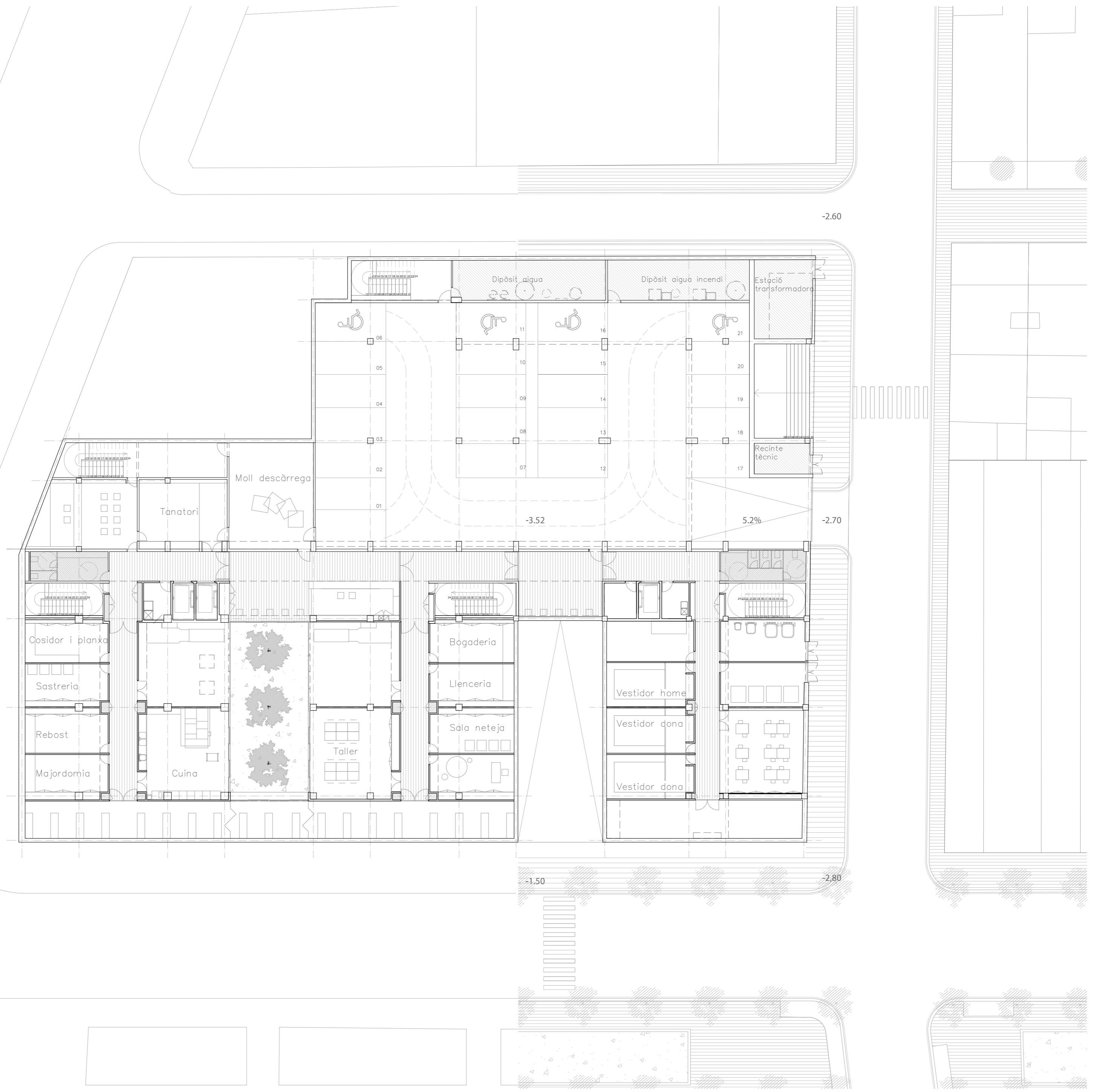
Planta pb-1 ( -3,52m)
