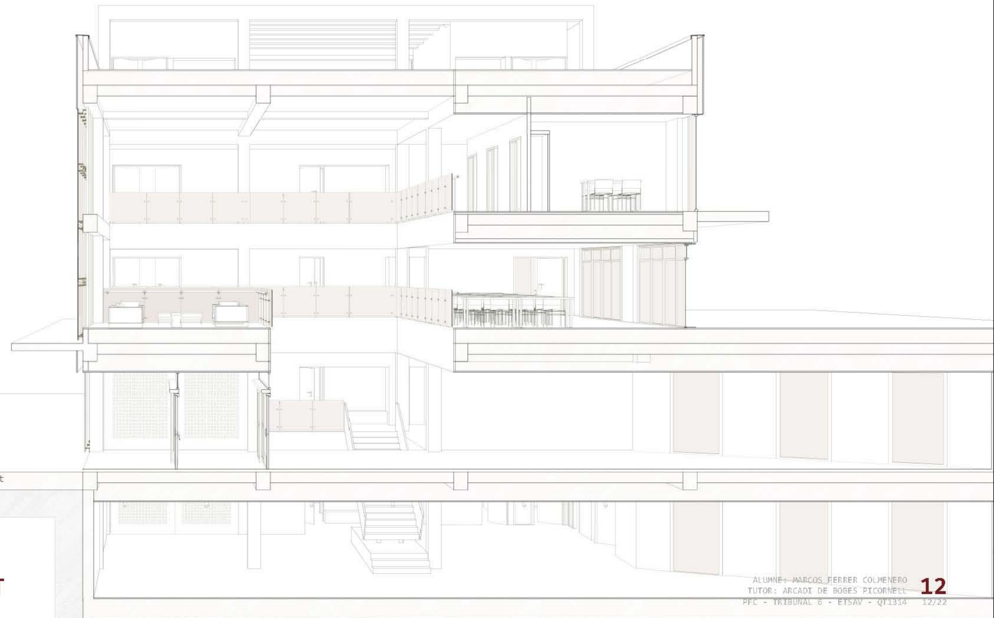
E2 Secció longitudinal equipament
