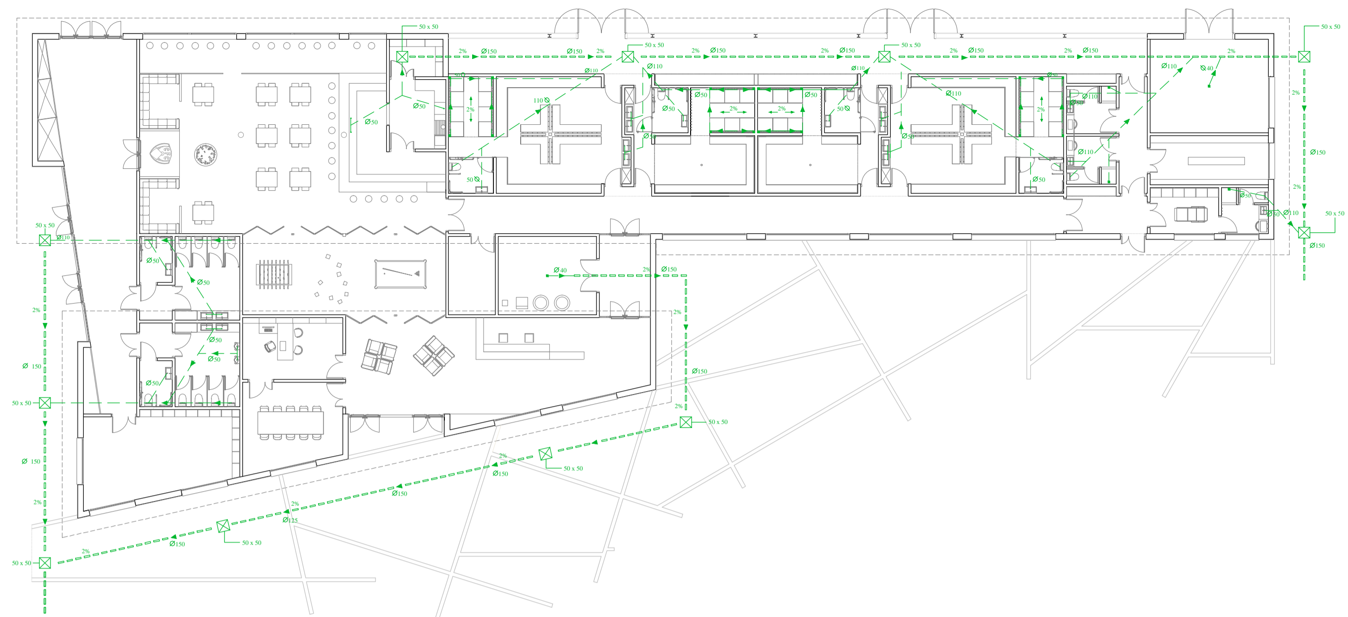
ESQUEMA SANEJAMENT ESCALA 1/200
