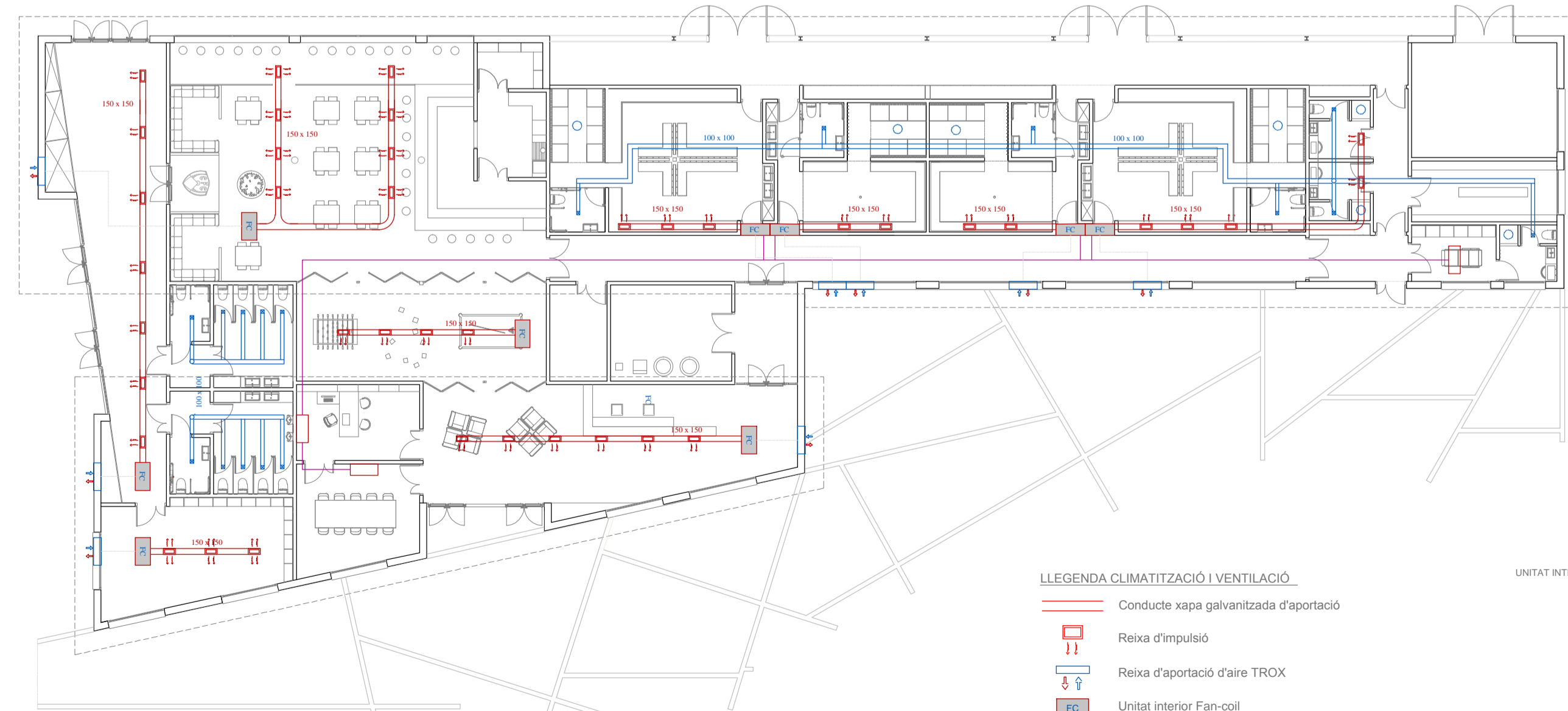
ESQUEMA CLIMATITZACIÓ I VENTILACIÓ ESCALA 1/200
