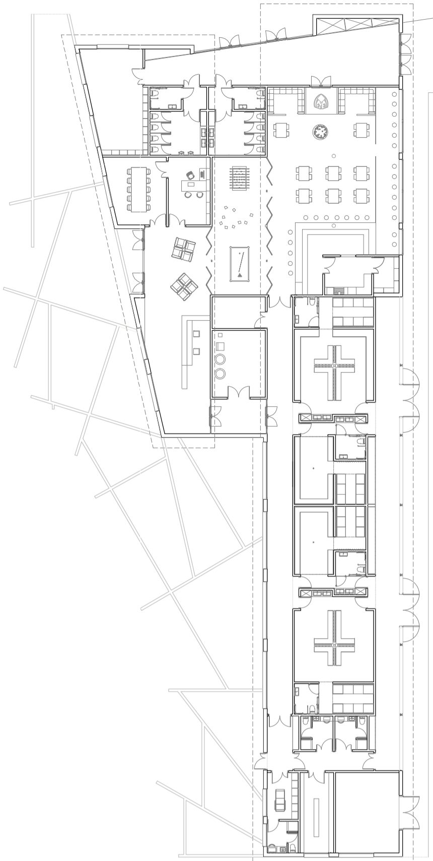
ESQUEMA SANEJAMENT CAMP ESCALA 1/300
