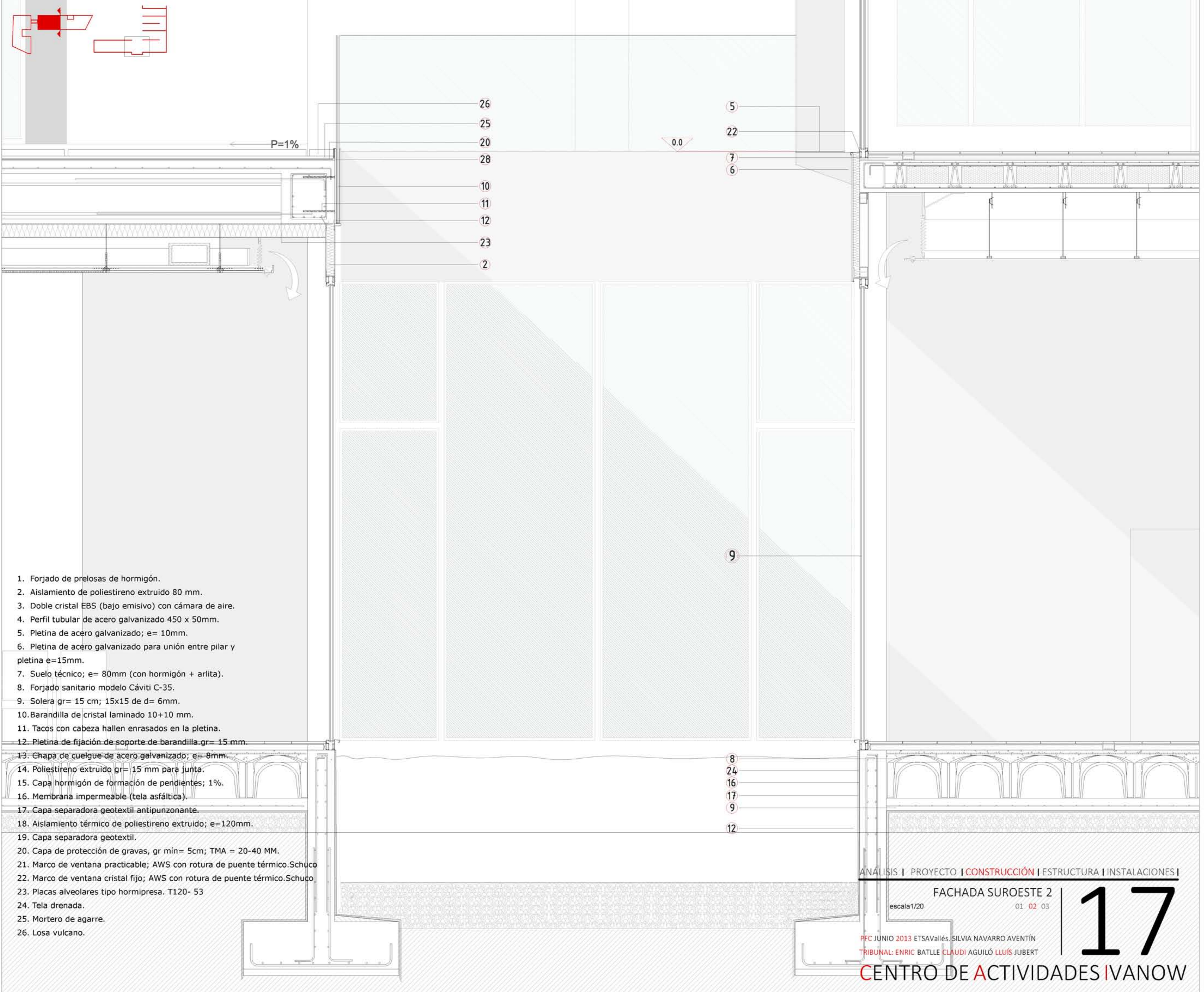
SECCIÓN 5 FACHADA SUROESTE E/ 1:20
