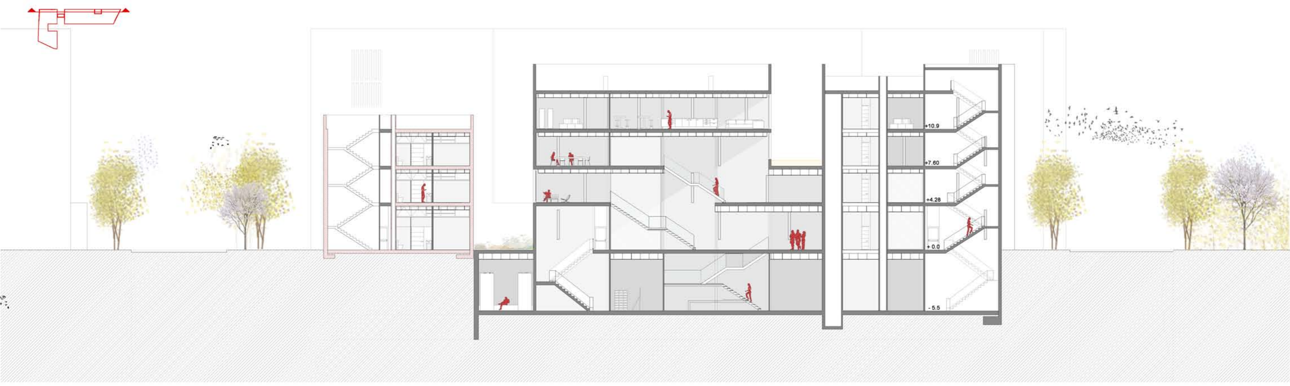
Sección 2 E/ 1:200
