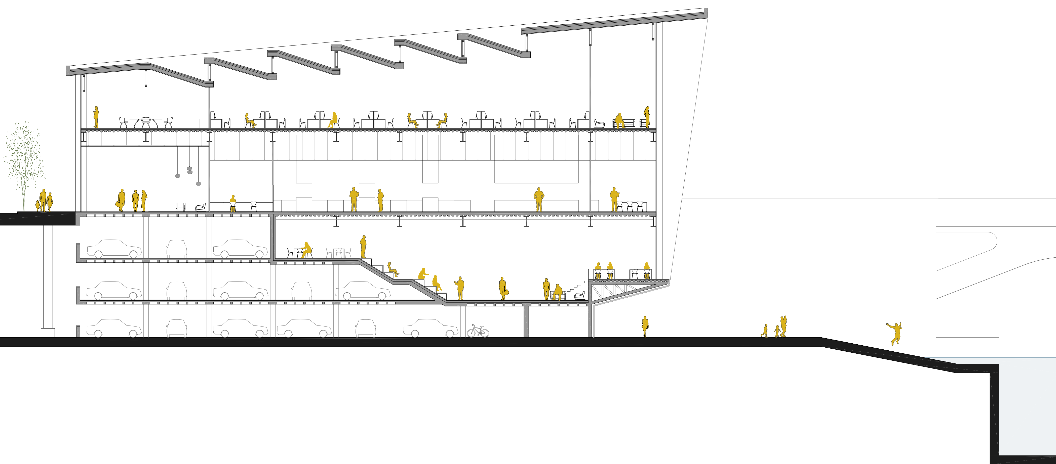
PLANTA BAIXA +9.60m | SECCIÓ LONGITUDINAL C ENTRE INVESTIGACIÓ E. 1:150
