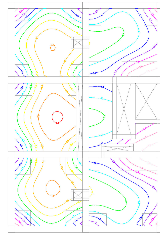
Planta Quinta Máx = 8.2 Min = 1.9
