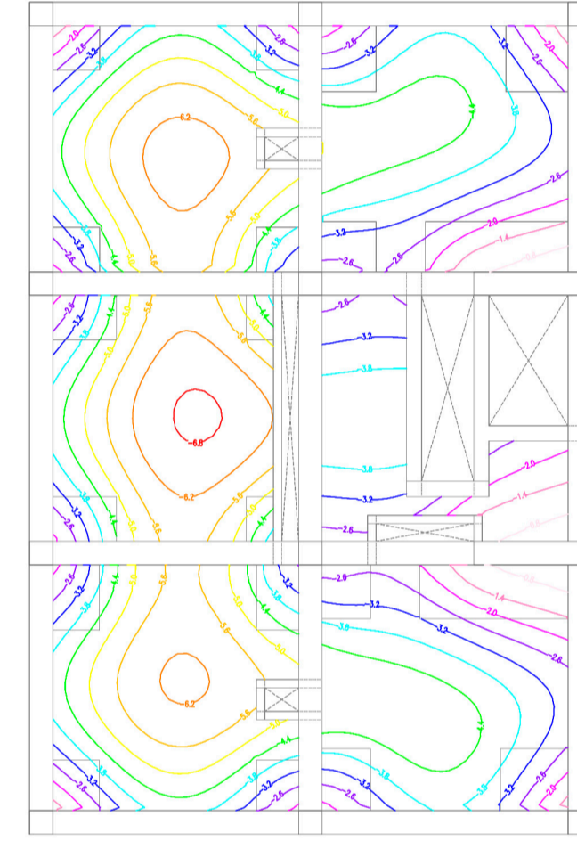
Planta Primera Máx = 6.8 Min = 0.8
