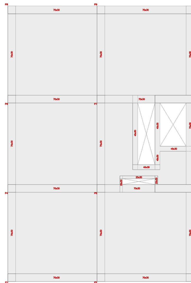
Plantas estructura PB
