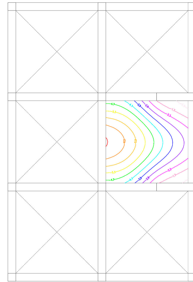
Planta Cubierta Máx = 6.5 Min = 1.7
