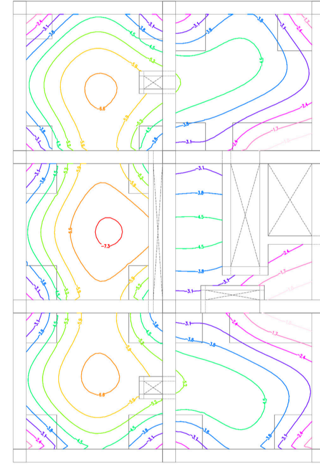
Planta Segunda Máx = 7.3 Min = 1.0
