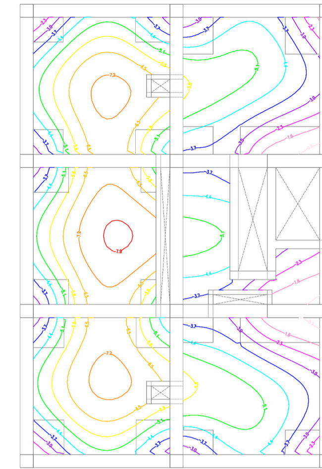
Planta Cuarta Máx = 7.9 Min = 1.6
