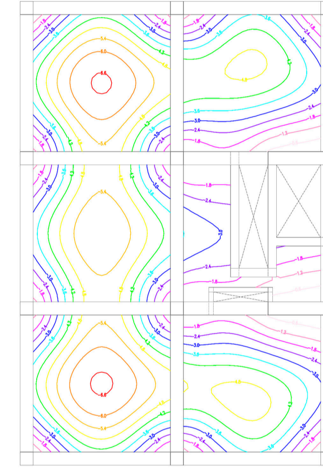
Planta Baja Máx = 6.6 Min = 0.6
