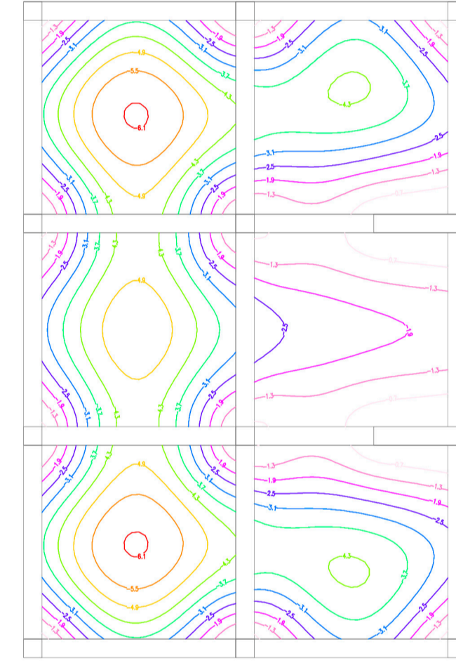
Planta Sotano Máx = 6.1 Min = 0.7
