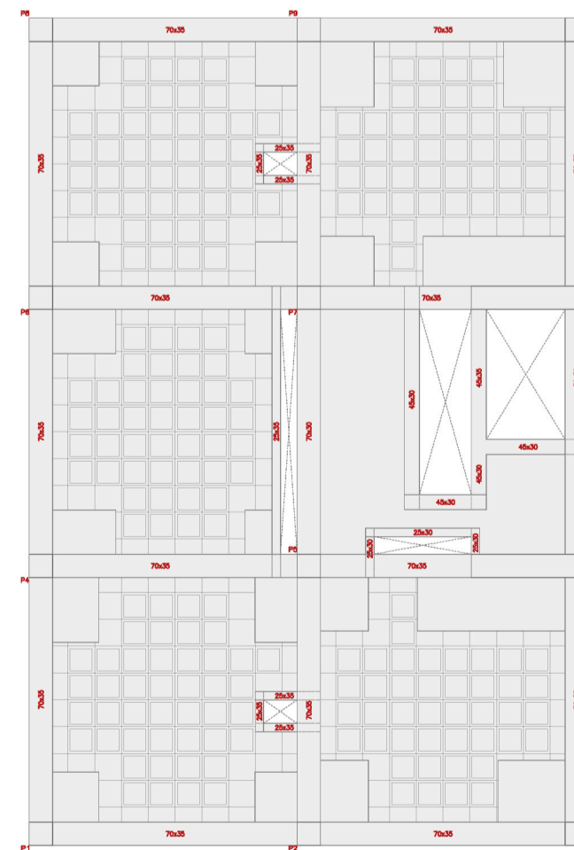
Plantas estructura de P1 hasta P8
