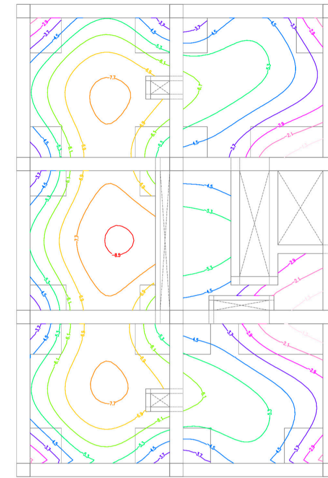
Planta Séptima Máx = 8.5 Min = 2.1
