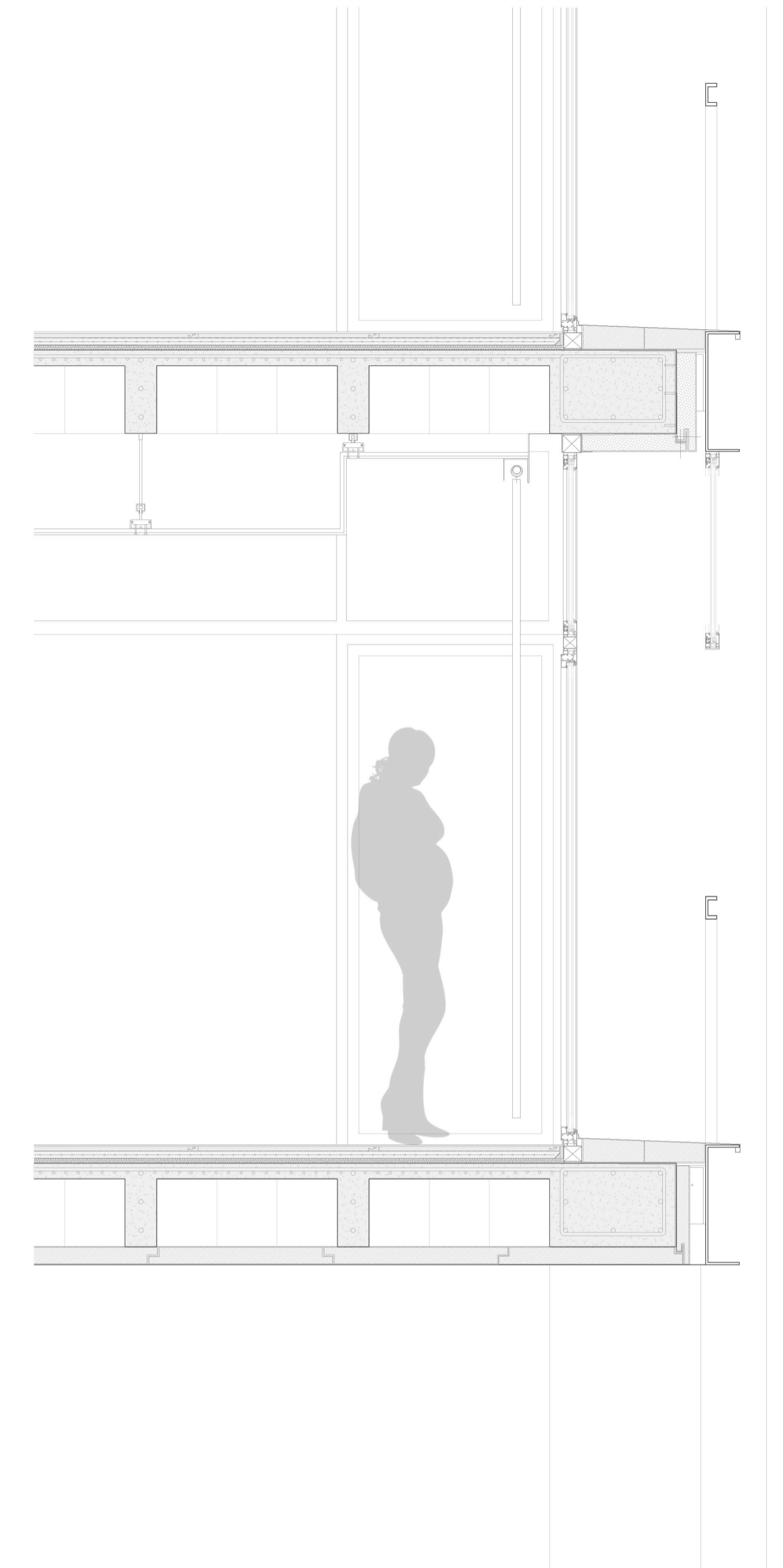
Vista de sección tipo del edificio caja
