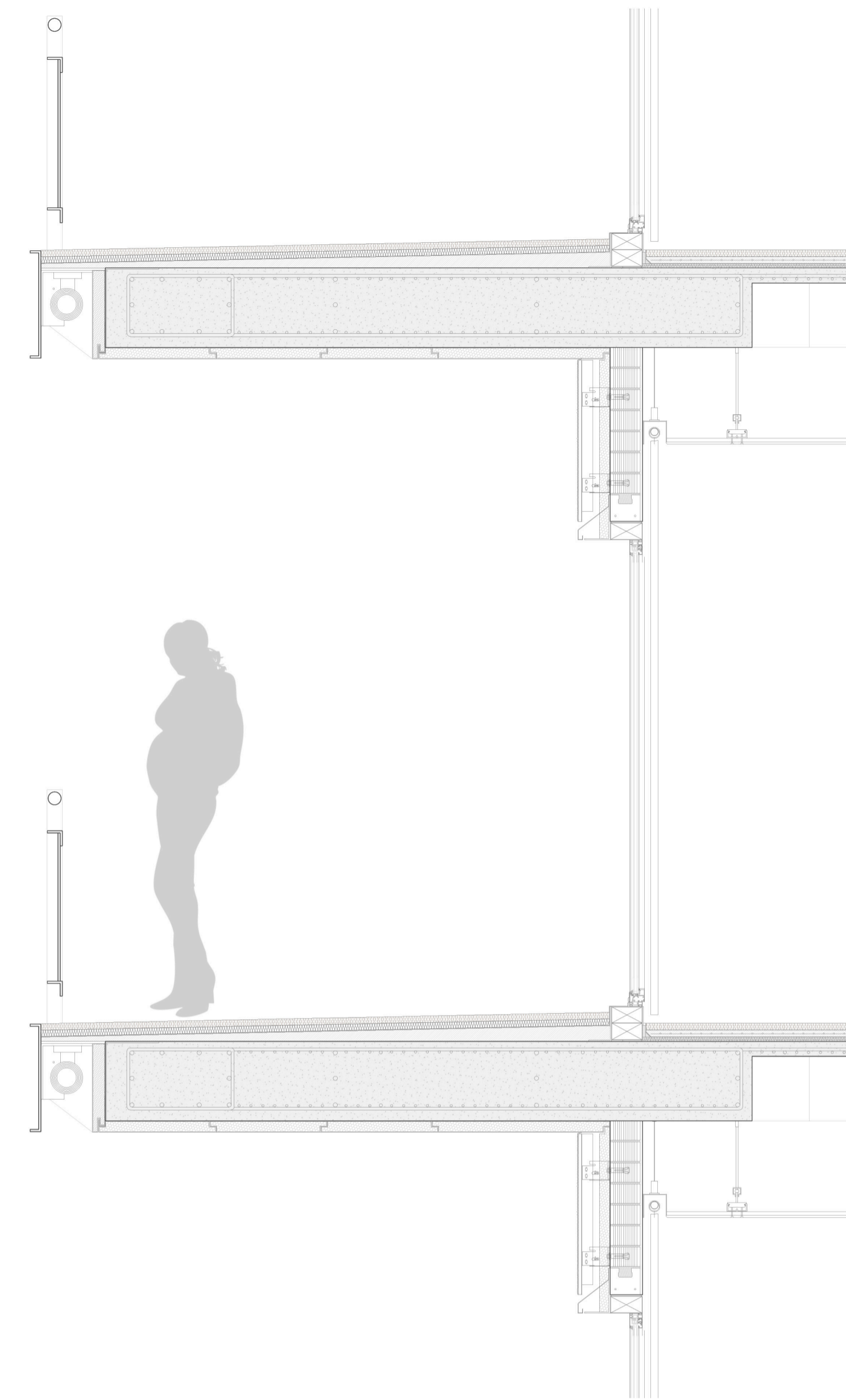
Vista de sección tipo del edificio barra
