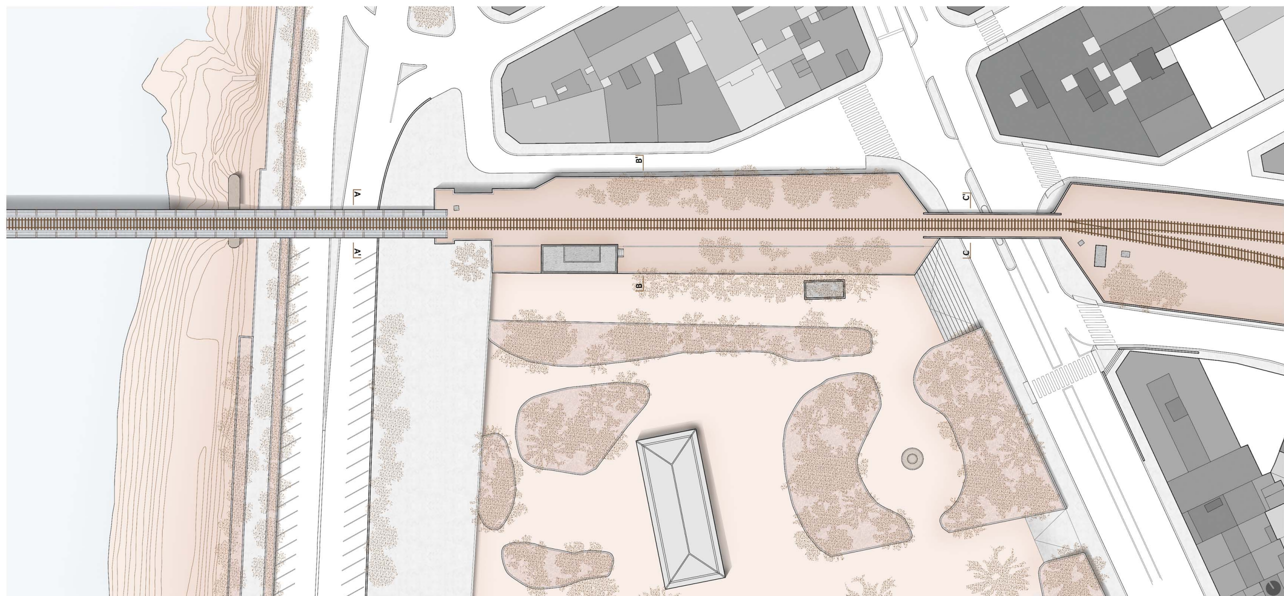
EMPLAZAMIENTO ESTADO ACTUAL E:1/500
