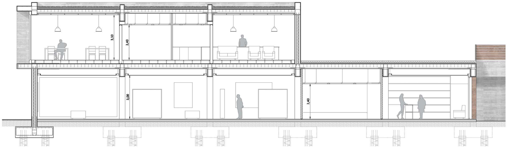
SECCIÓN B-B' E:1/100
