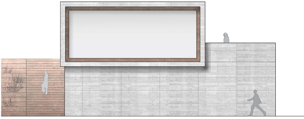
ALZADO OESTE E:1/100
