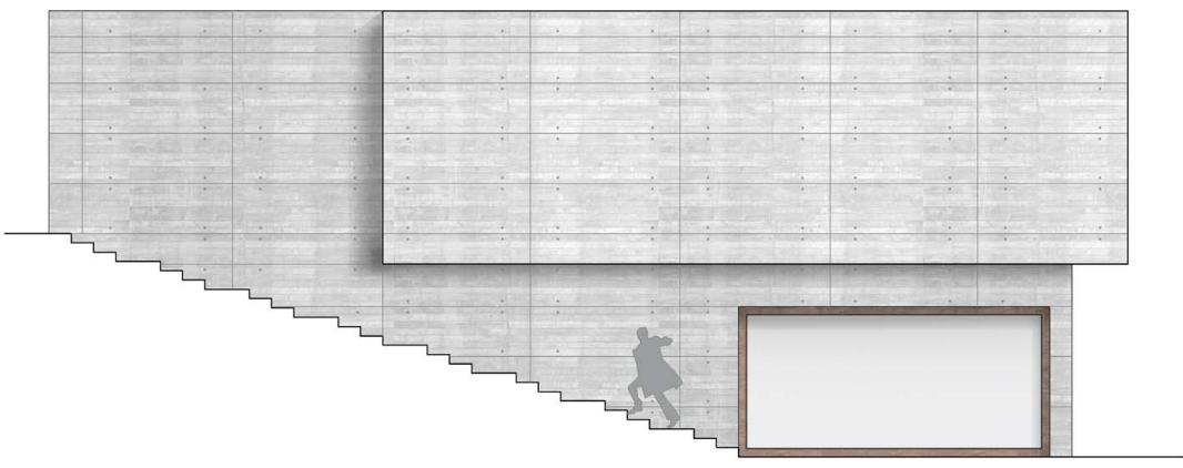
ALZADO NORTE ENSANCHE E:1/100
