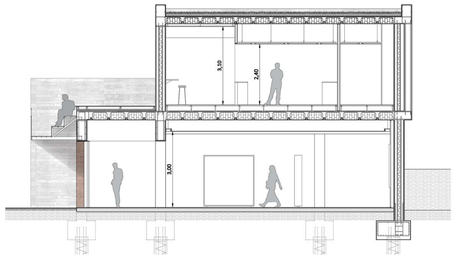
SECCIÓN A-A' E:1/100
