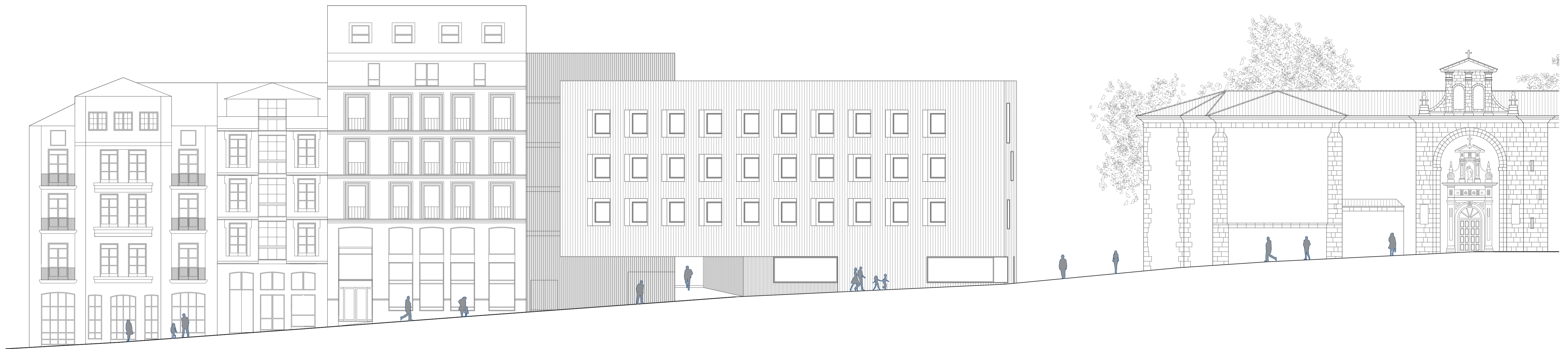
ALZADO NORTE E:1.150
