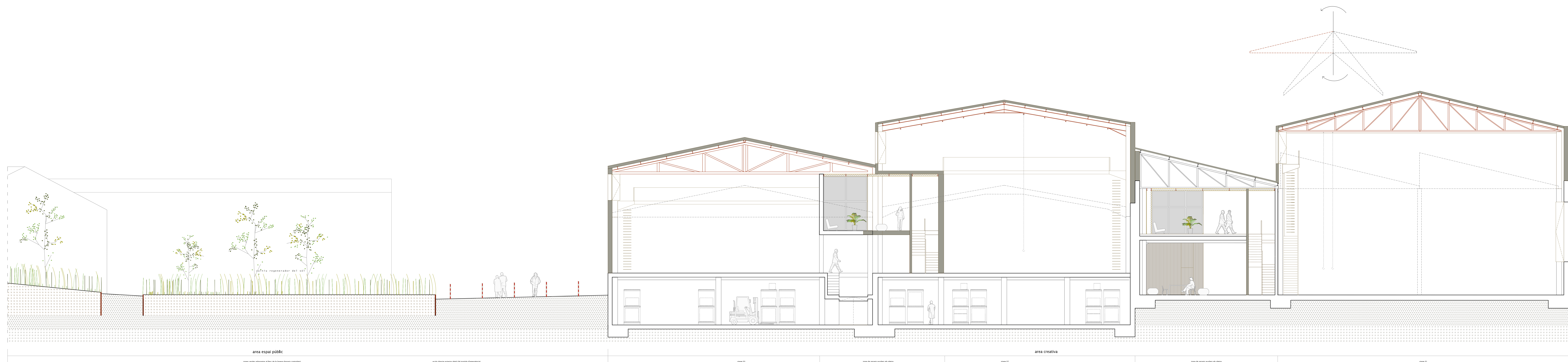
Secció transversal 02
