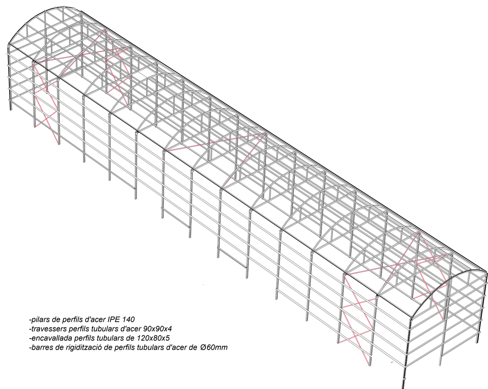
estructura de gran hivernacle
