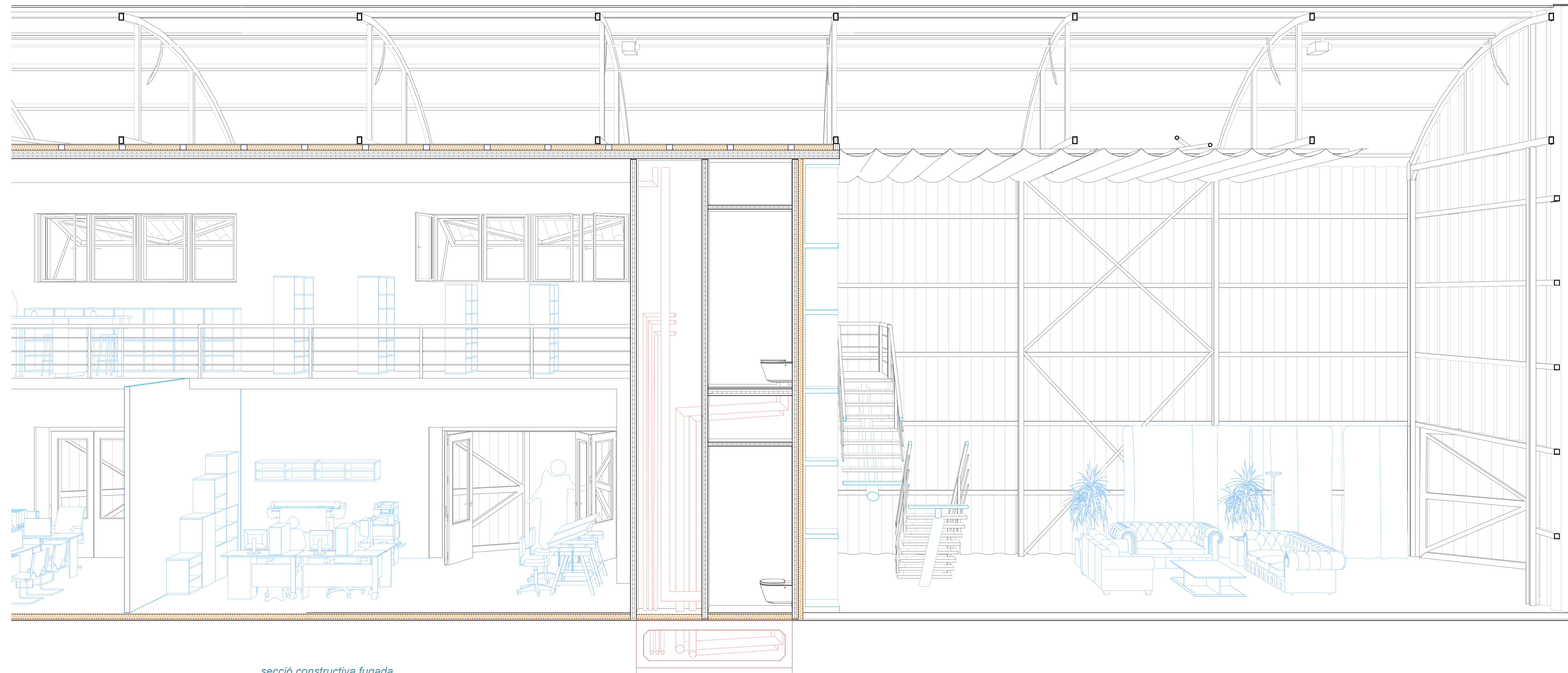
secció constructiva fugada e1:30
