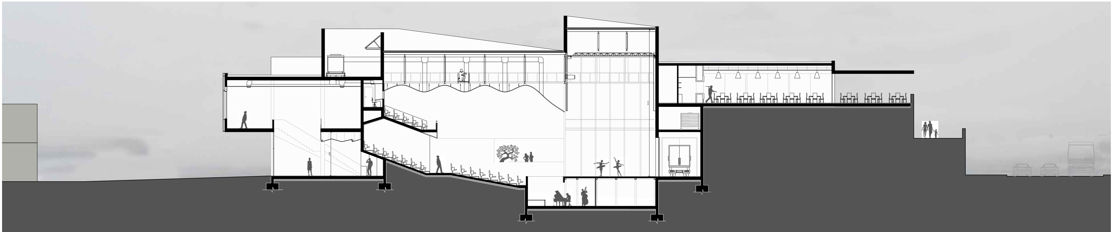
SECCIÓ B-B
