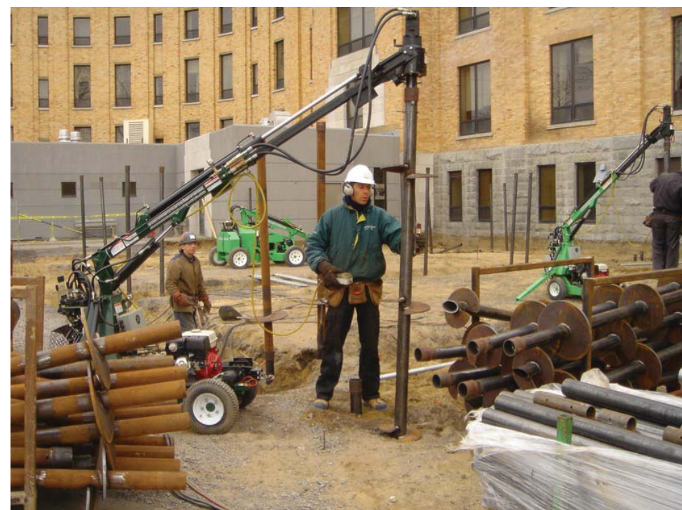
Sistema Fonamentació
