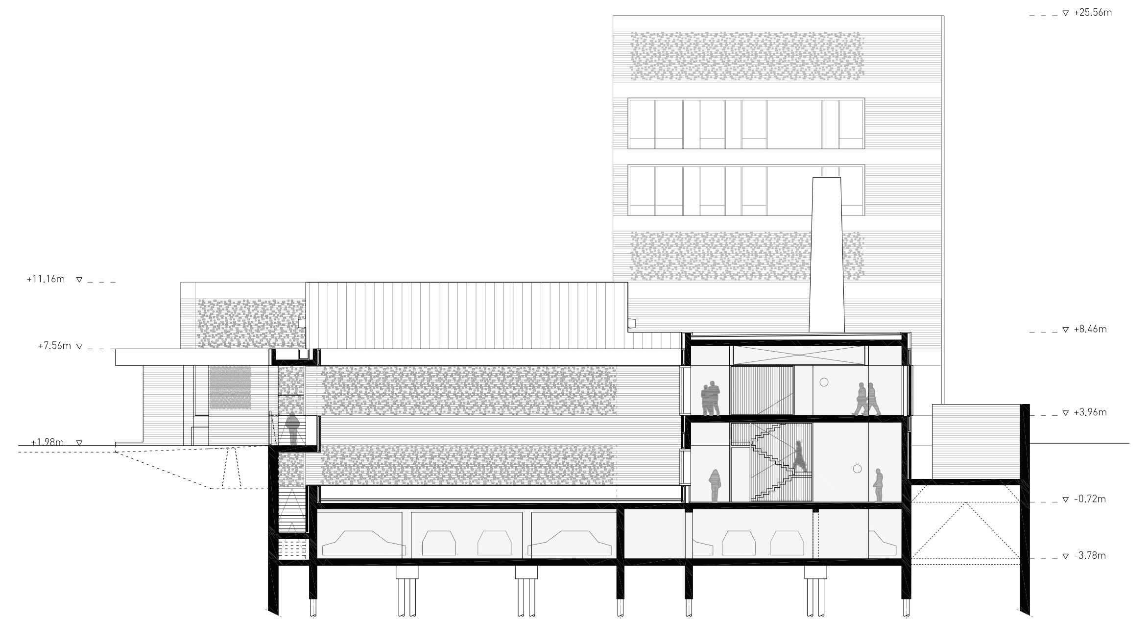
Secció Transversal L-L' 1:200 Vista per pati de servei, nucli vertical de cuines i magatzems
