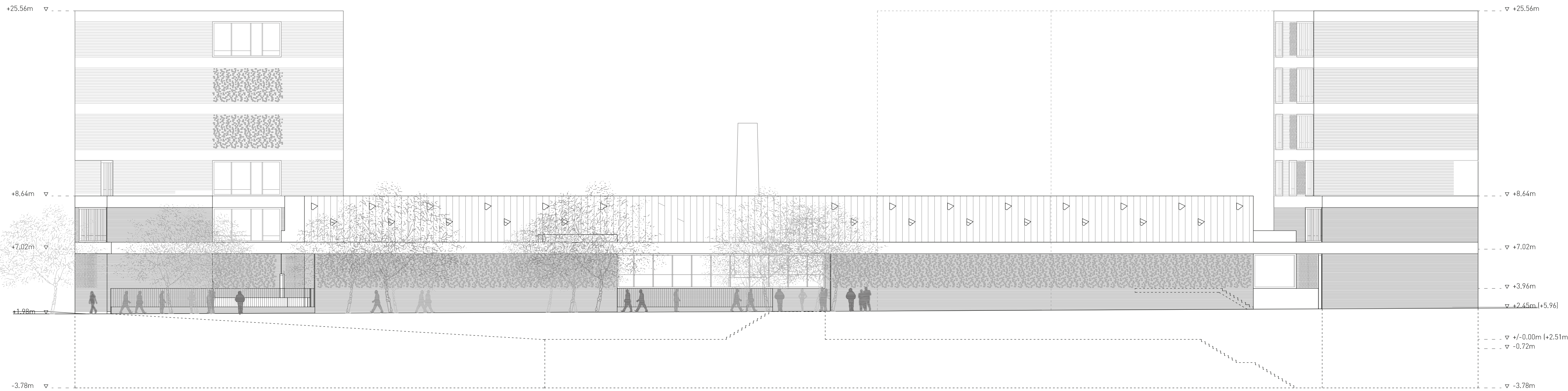
Alçat Sud (E-E') 1:200 Alçat carrer Marroc Accés principal públic, façana sud
