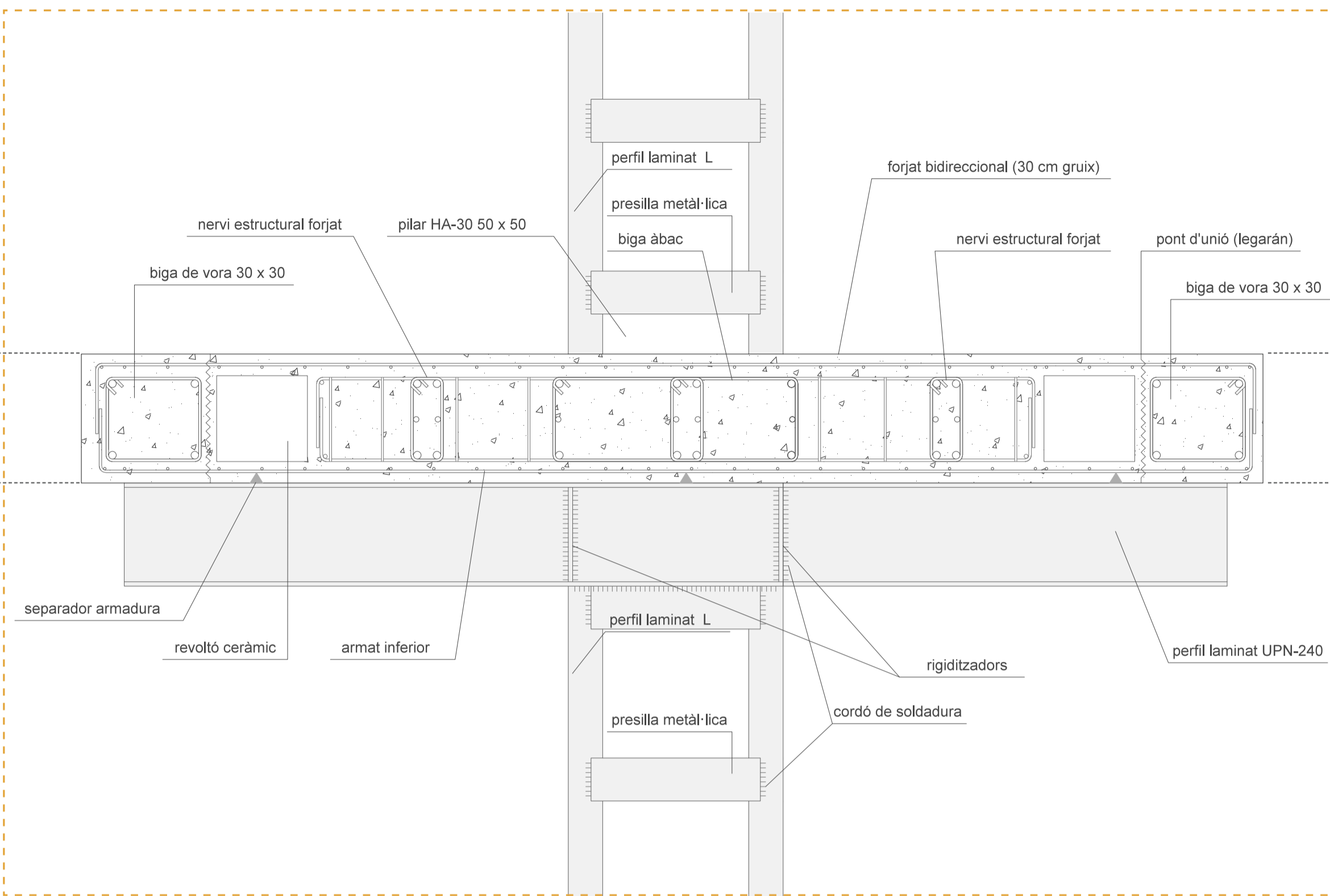
• Detall 2 e: 1/10
