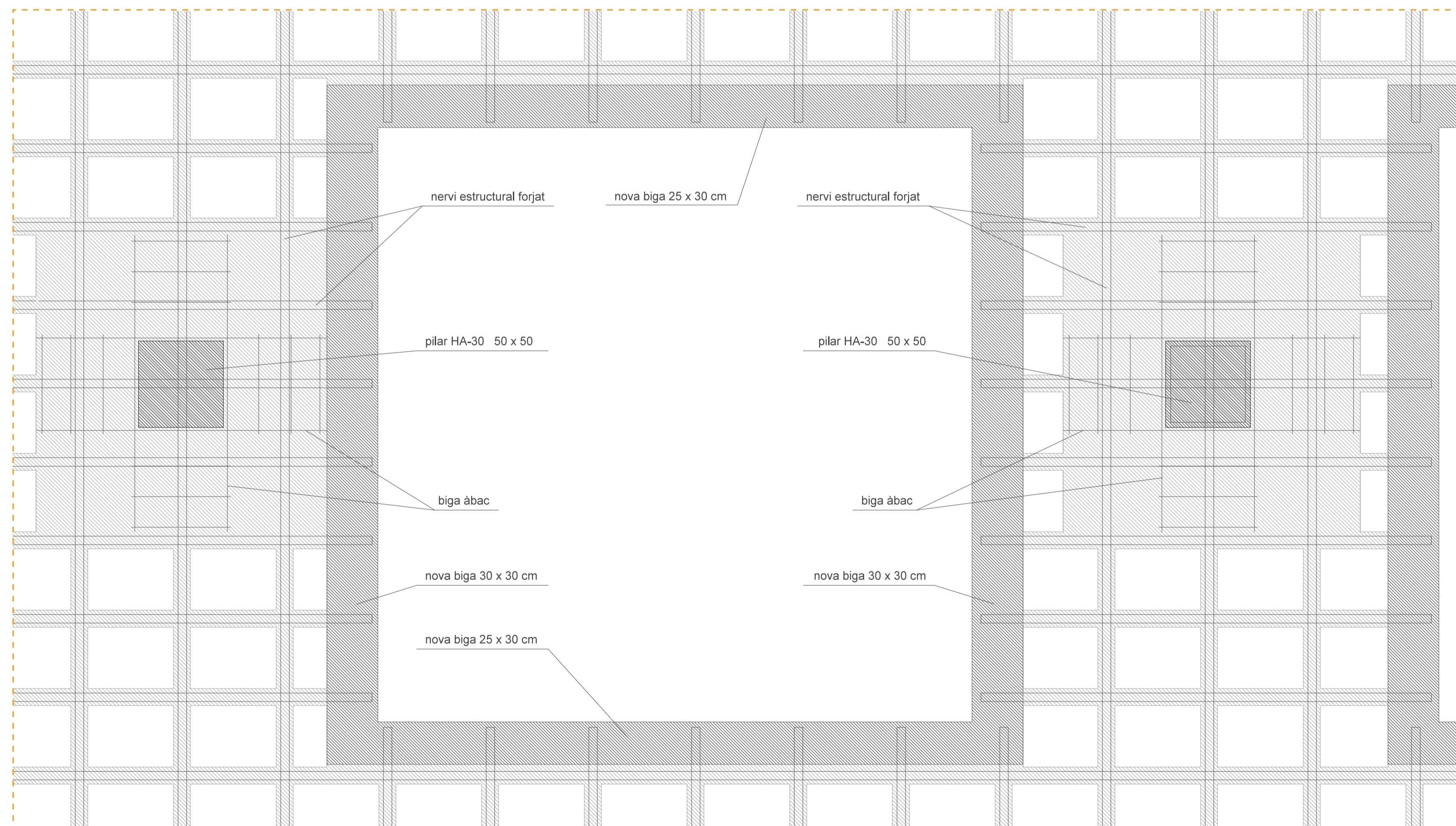
• Detall 3 e: 1/20
