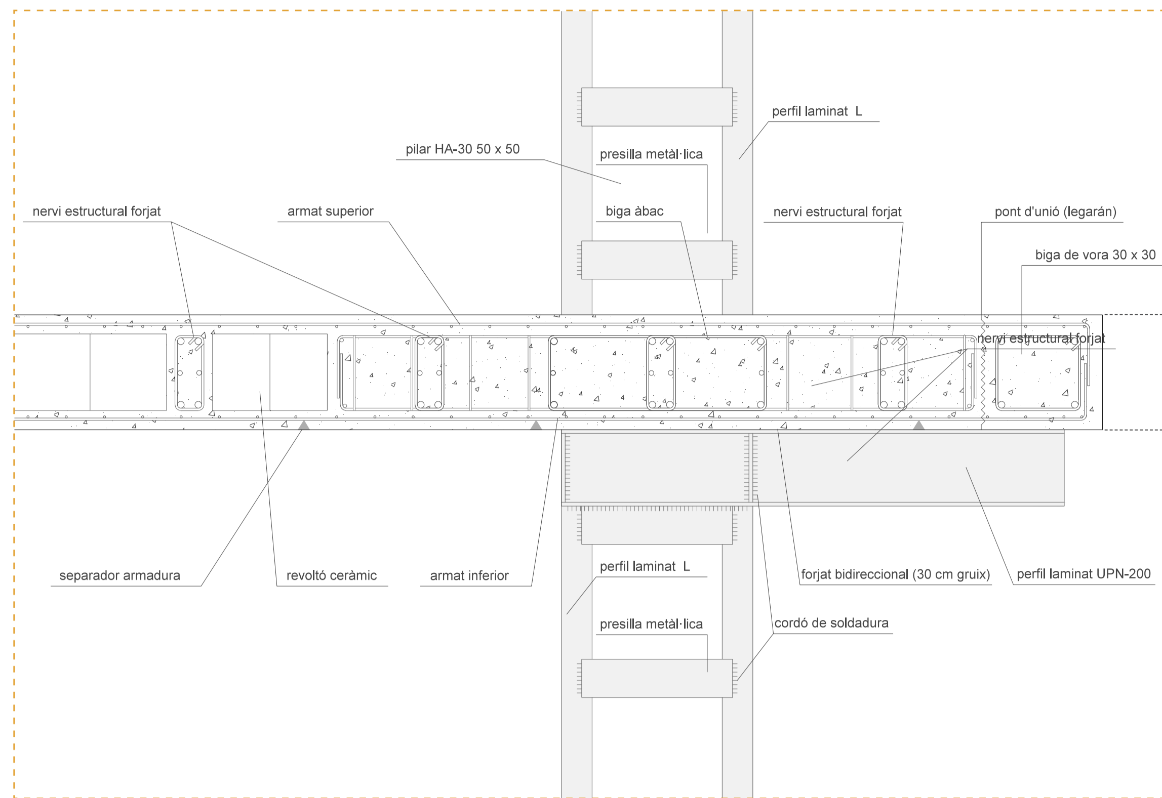
• Detall 1 e: 1/10
