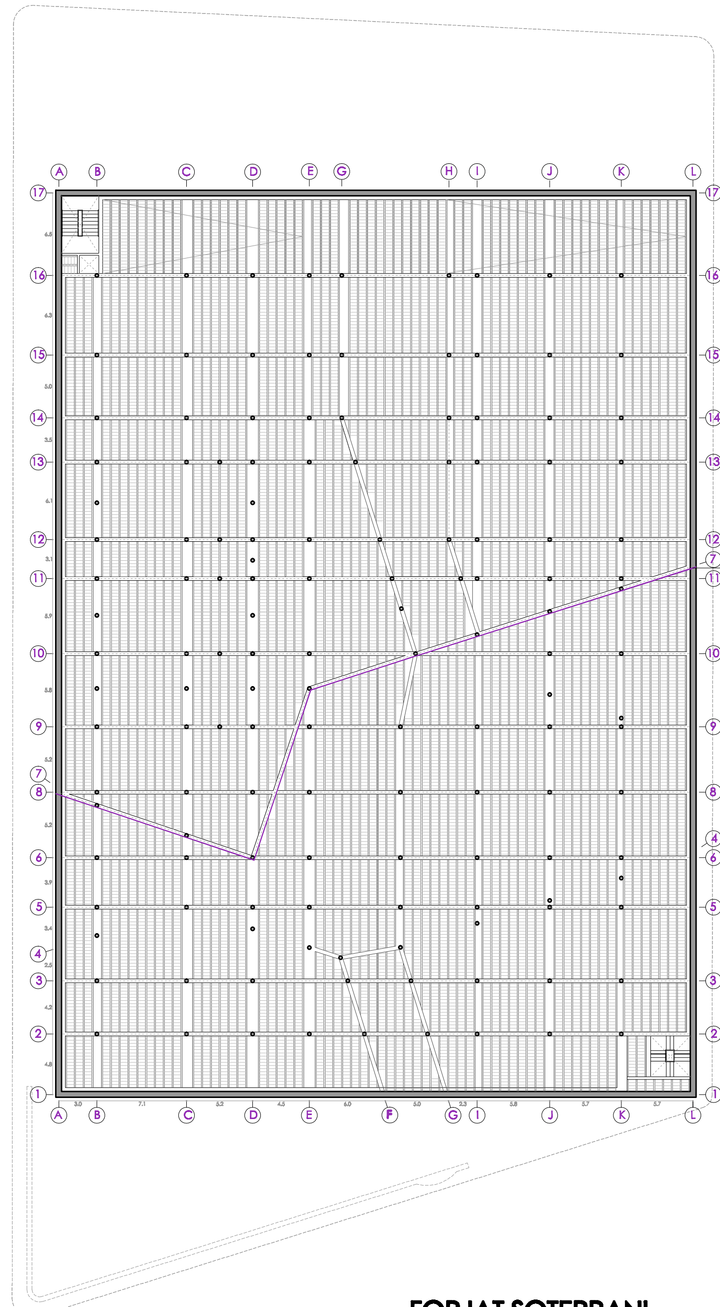
FORJAT SOTERRANI (+54.00)
