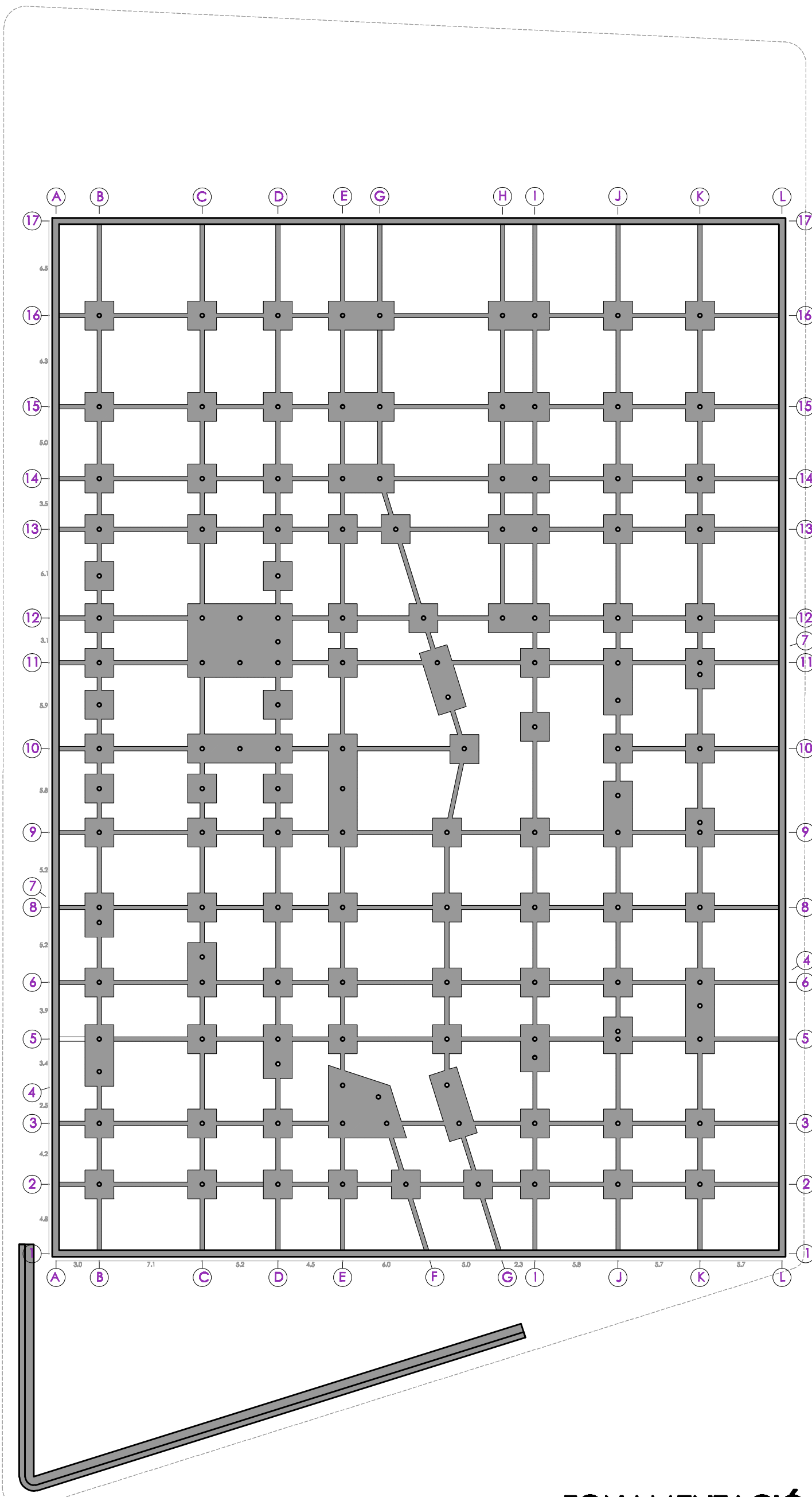
FONAMENTACIÓ
