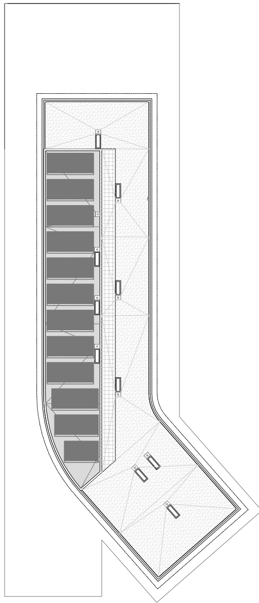
PLANTA BADALOT (+41.40) | -PLAQUES SOLARS D'ALT RENDIMENT
