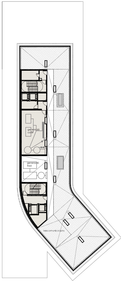
PLANTA COBERTA (+38.70)
