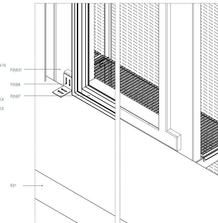
SISTEMA CONSTRUCTIU I DE SUPORT PELS PANELLS PREFABRICATS DE FORMIGÓ
