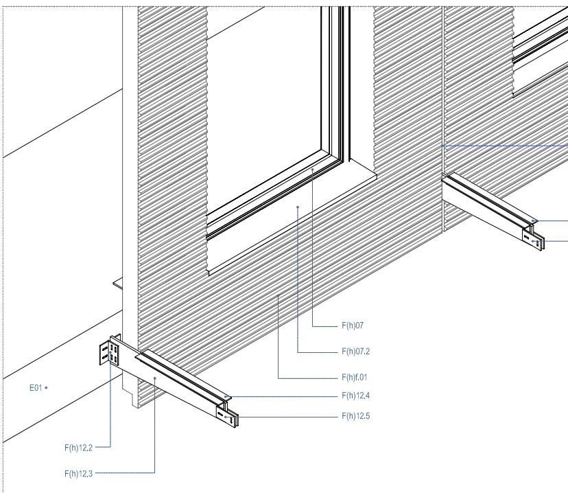
SISTEMA CONSTRUCTIU I DE SUPORT PEL DÉPLOYÉ
