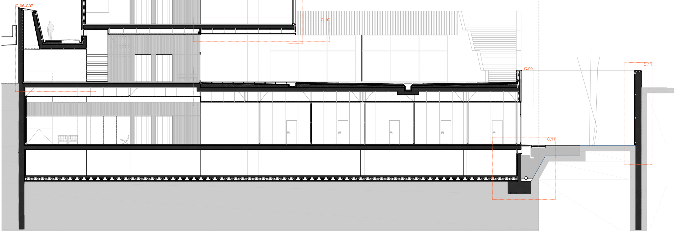
Secció transversal 2: INDEX DETAILS
