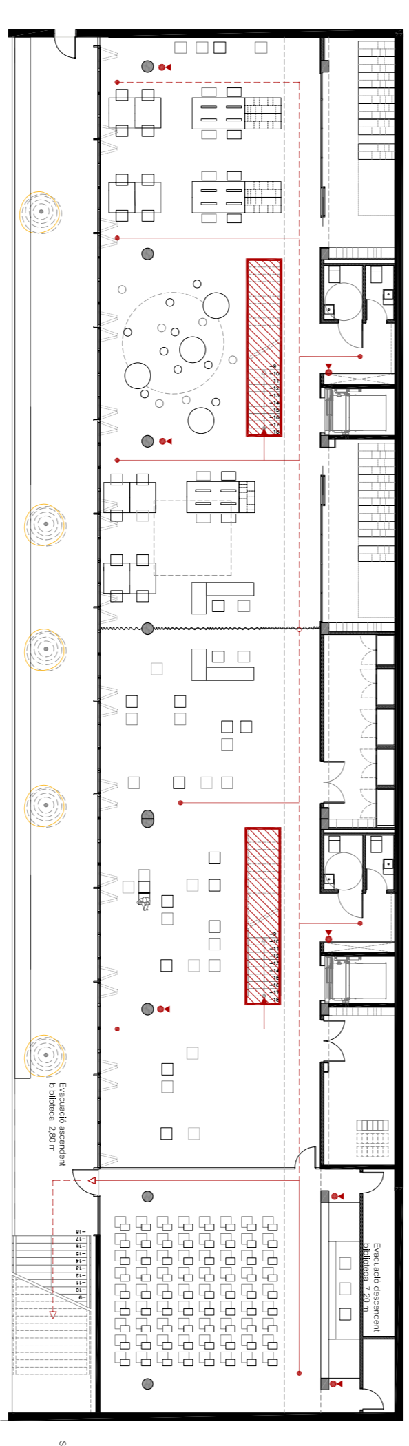
PLANTA SOTERRANI
