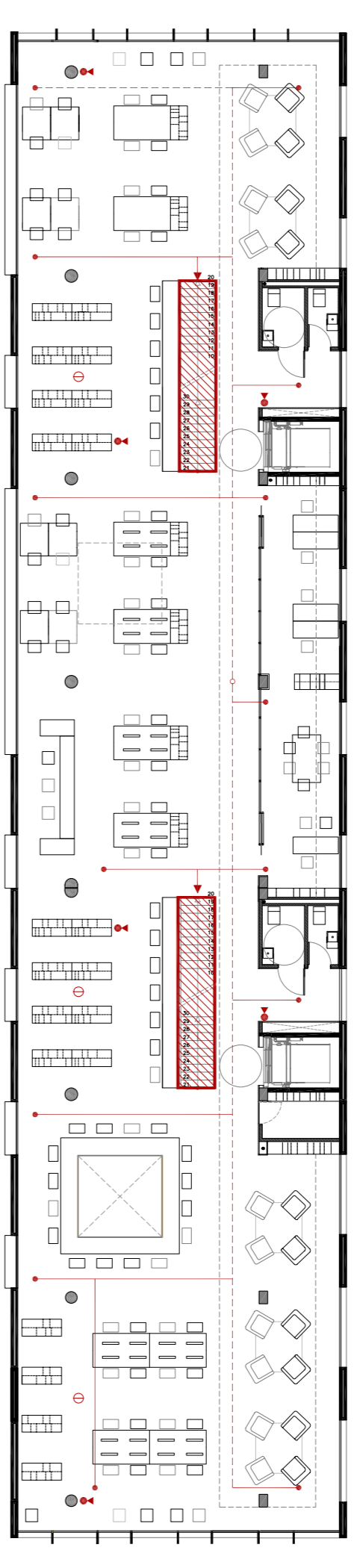
PLANTA PRIMERA
