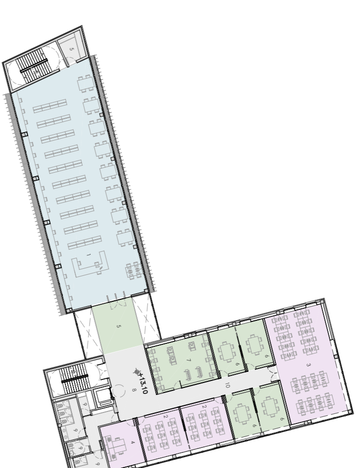
PLANTA P3 cota forjado +13.10
