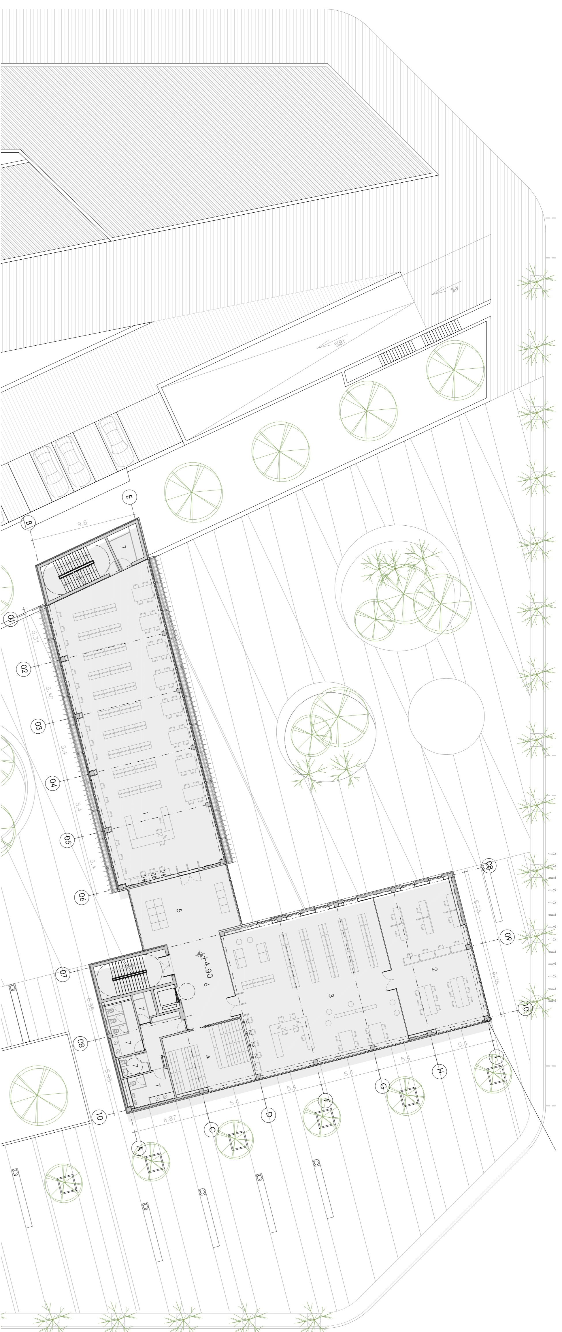
PLANTA P1 cota forjado +4.90
