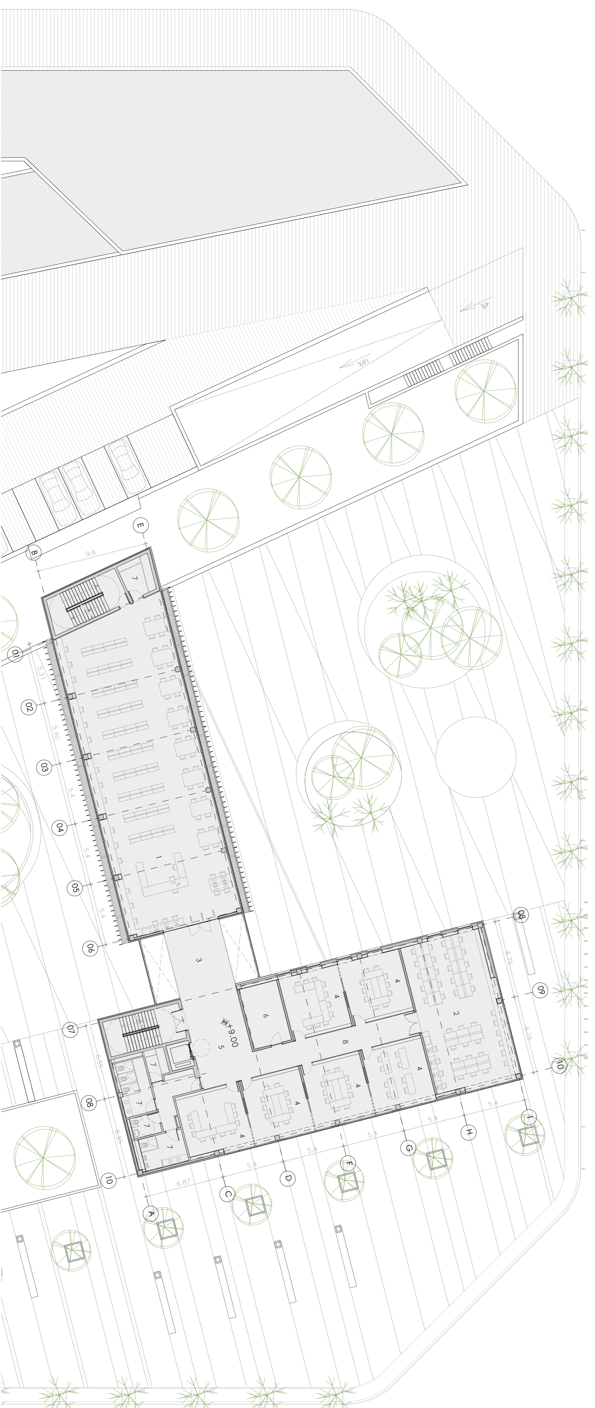
PLANTA P2 cota forjado +9.00
