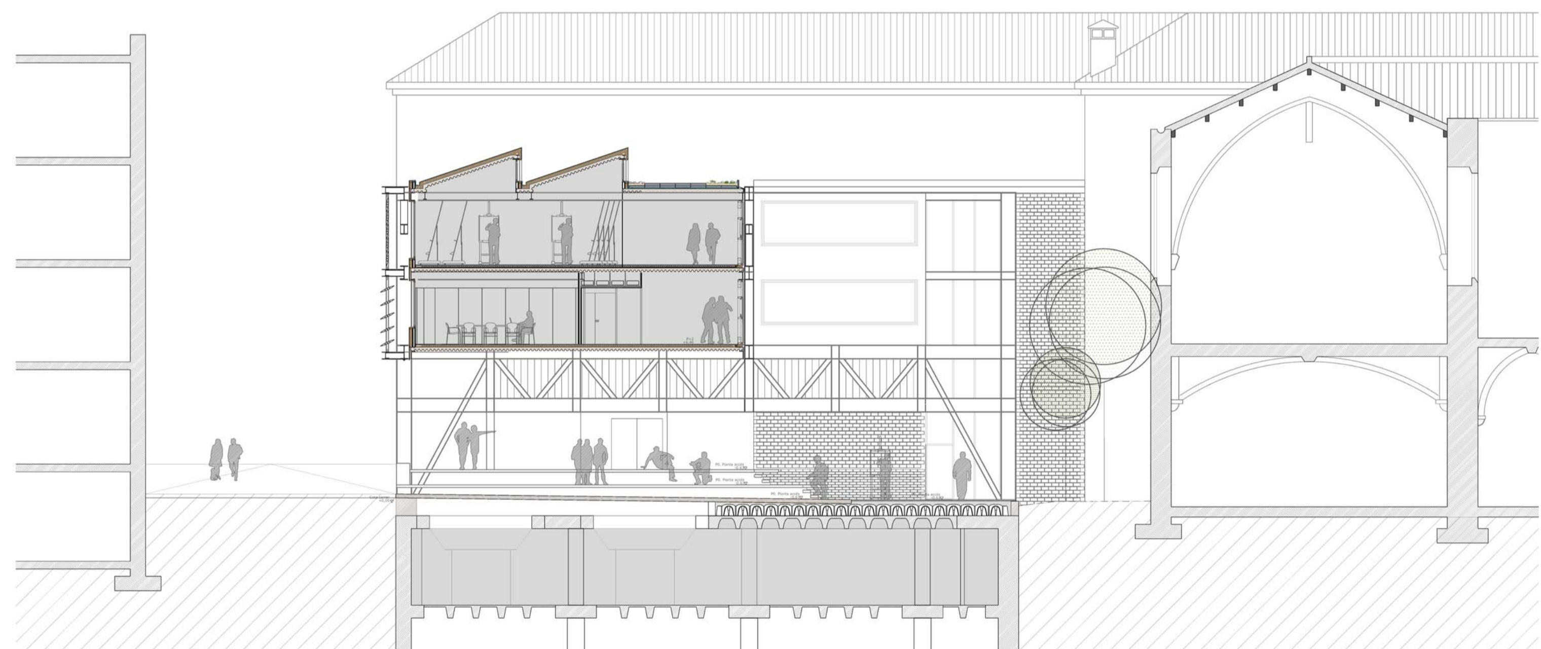
secció_A-A'
