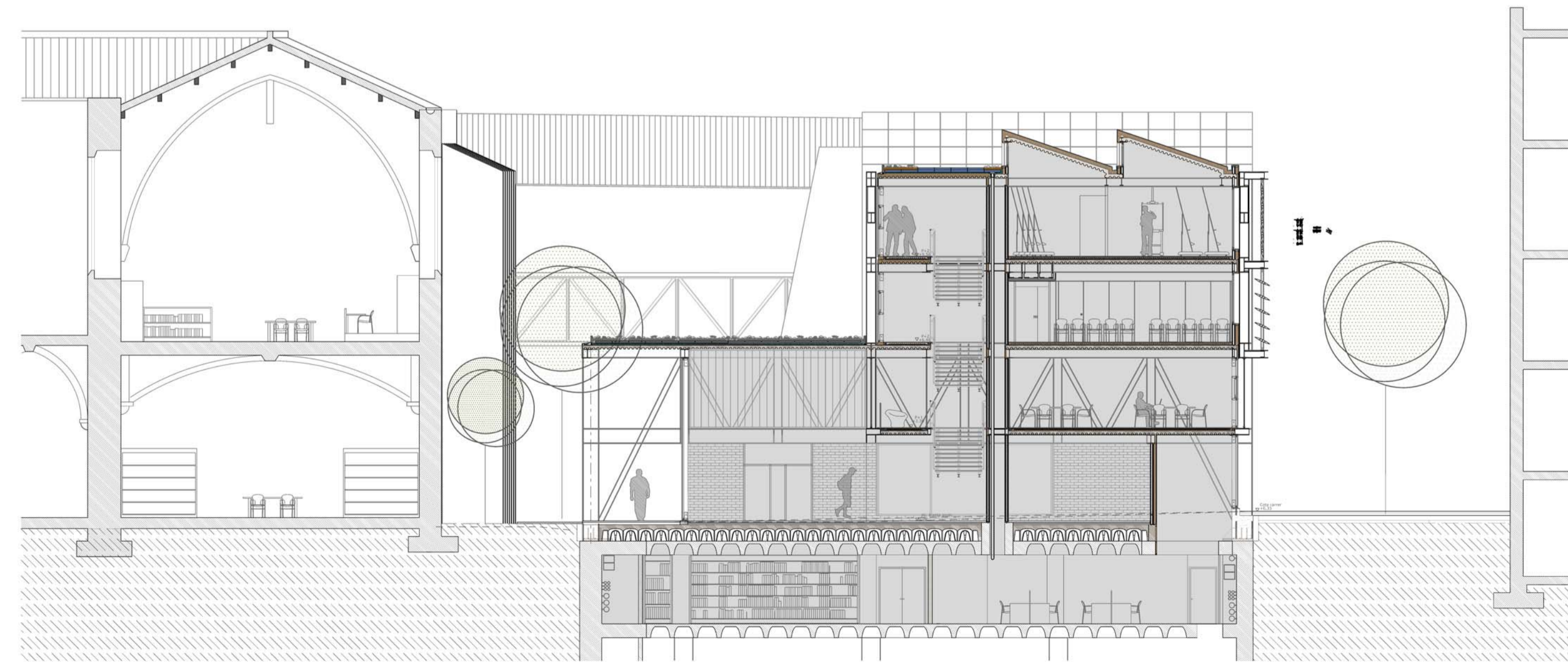
secció_B-B'
