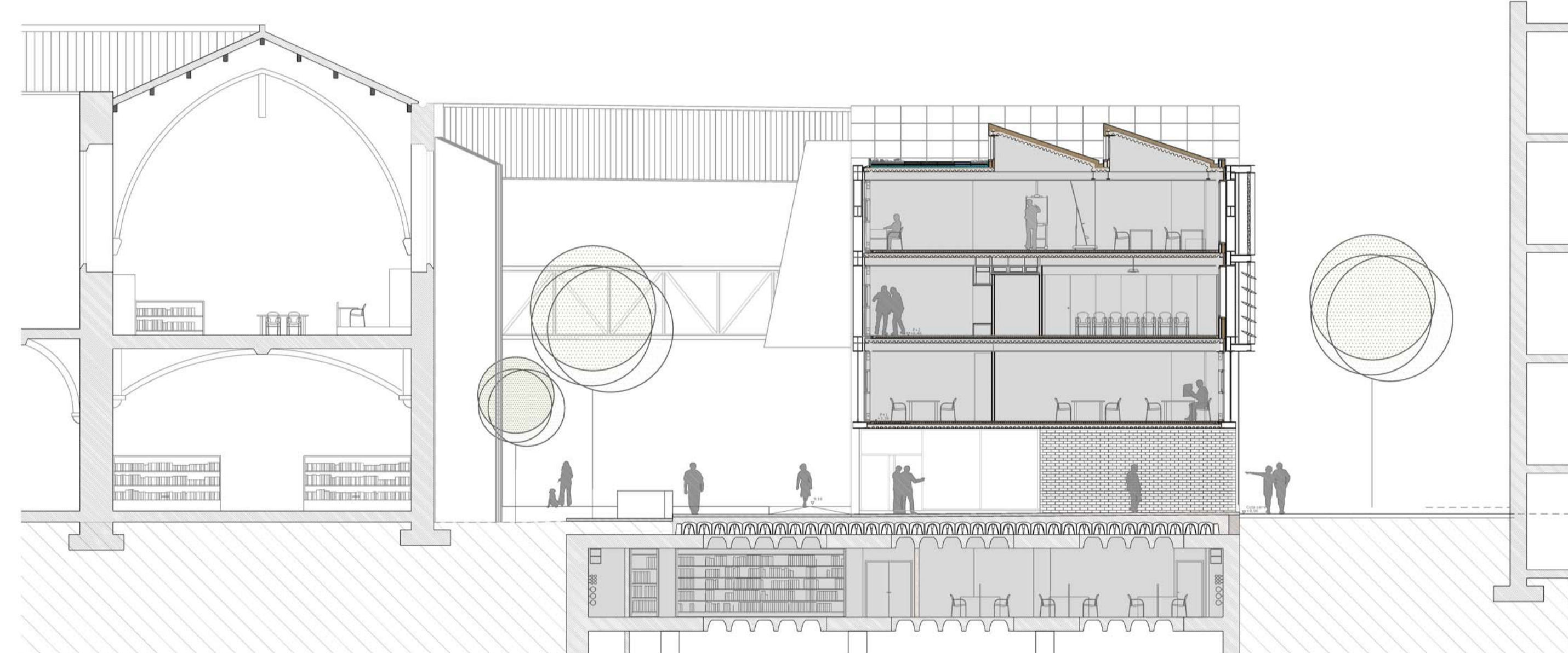
secció_C-C'
