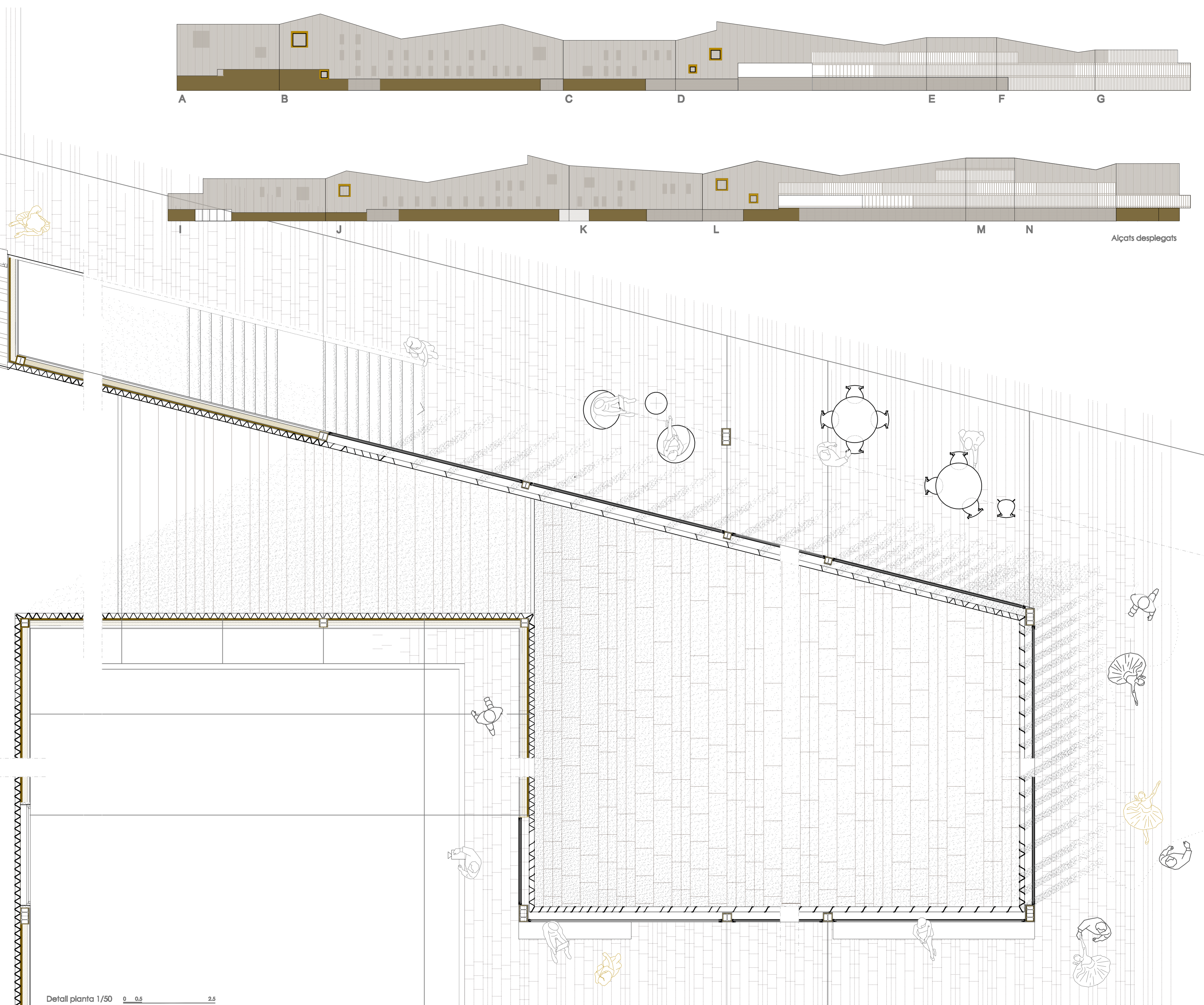
Detall planta 1/50 0 0.5 2.5
